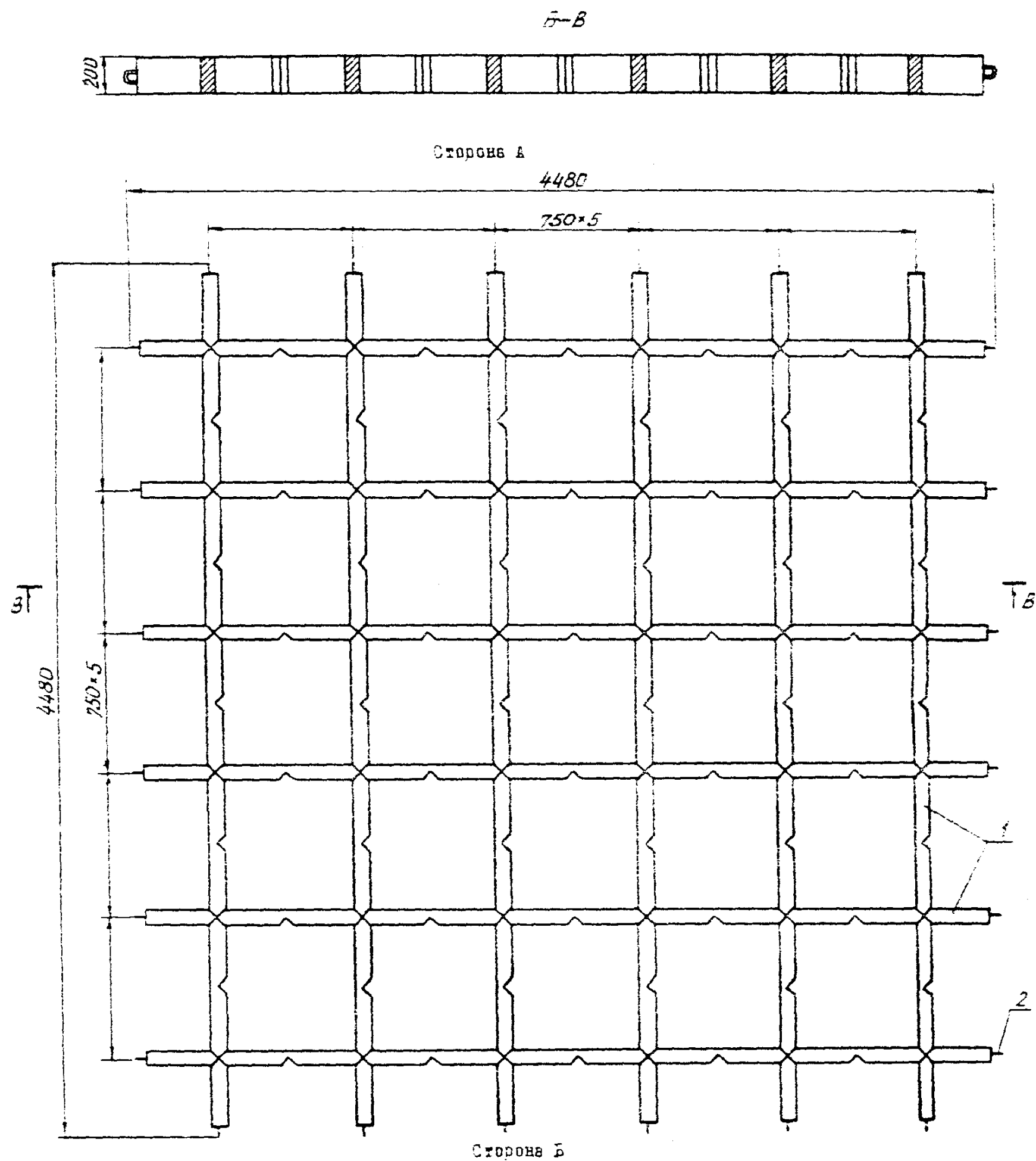
Рис. 4. Блок решетчатого покрытия: 1- гибкая железобетонная гирлянда сечением 20,0×7,5 см; 2- петли для стыкования диаметром 12 мм, длиной 484 мм
