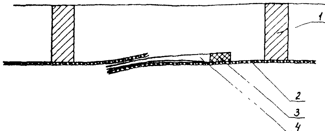
Рис. 6. Обратный клапан:
