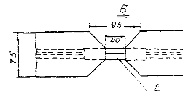
Рис. 5. Гирлянда железобетонного решетчатого покрытия: 1 — петли для стыкования диаметром 12 мм, длиной 484 мм; 2 — полиэтиленовая оболочка толщиной 2 мм, длиной 115 мм; 3 — пазы линейных шарниров
