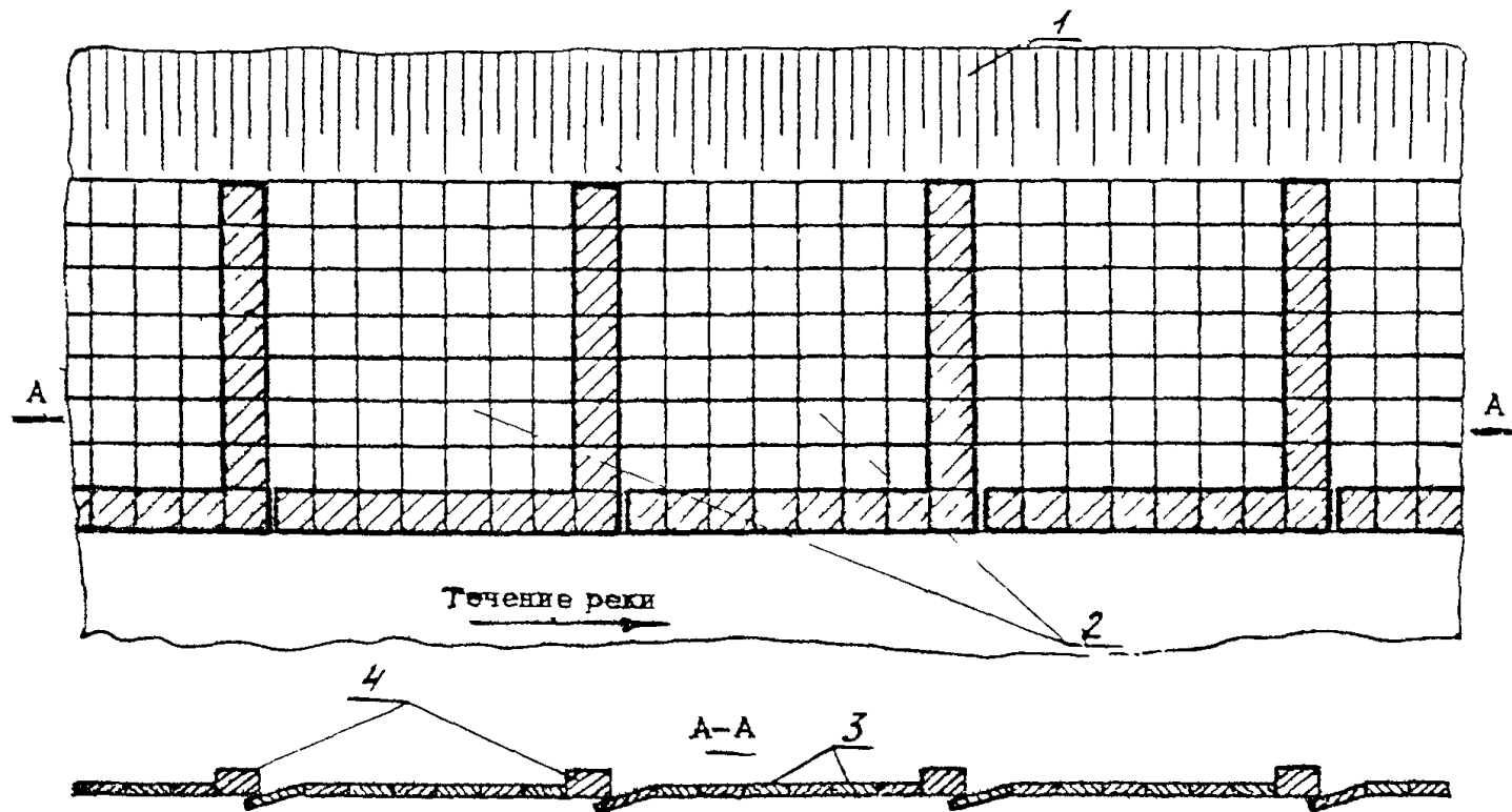
Рис. 3. Схема раскладки плит покрытия:
