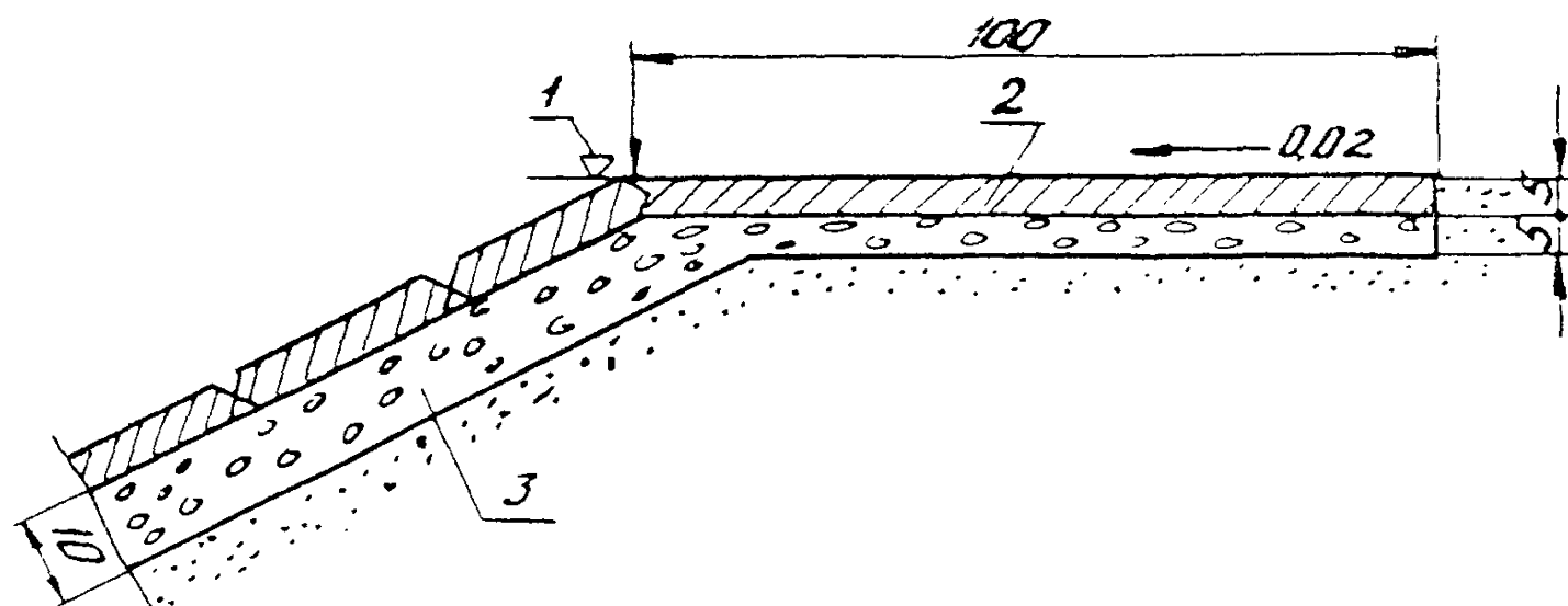
Рис. 8. Сопряжение покрытия с бровкой откоса:
