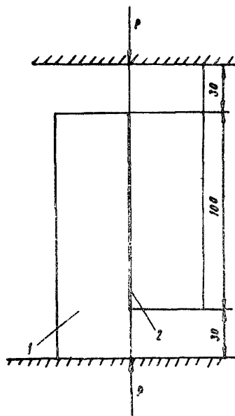
Рис.3. Схема для определения сцепления герметизирующих материалов с бетоном : 1-бетонная балочка 40х40х160мм; 2-мастика 0,5х20х100мм
