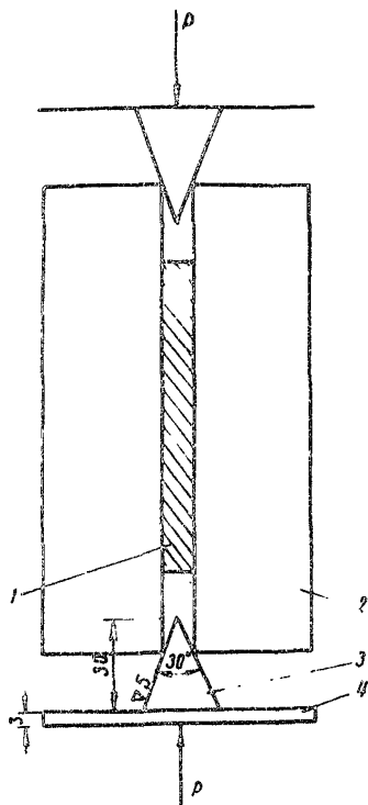
Рис.2. Испытание образца-шва на гидравлическом прессе : 1-мастика 8x20x100мм; 2-бетонная балочка 40x40x160мм ; 3-шип с конусом 30^{\circ} ; 4-металлическая пластина 3x40x90мм
