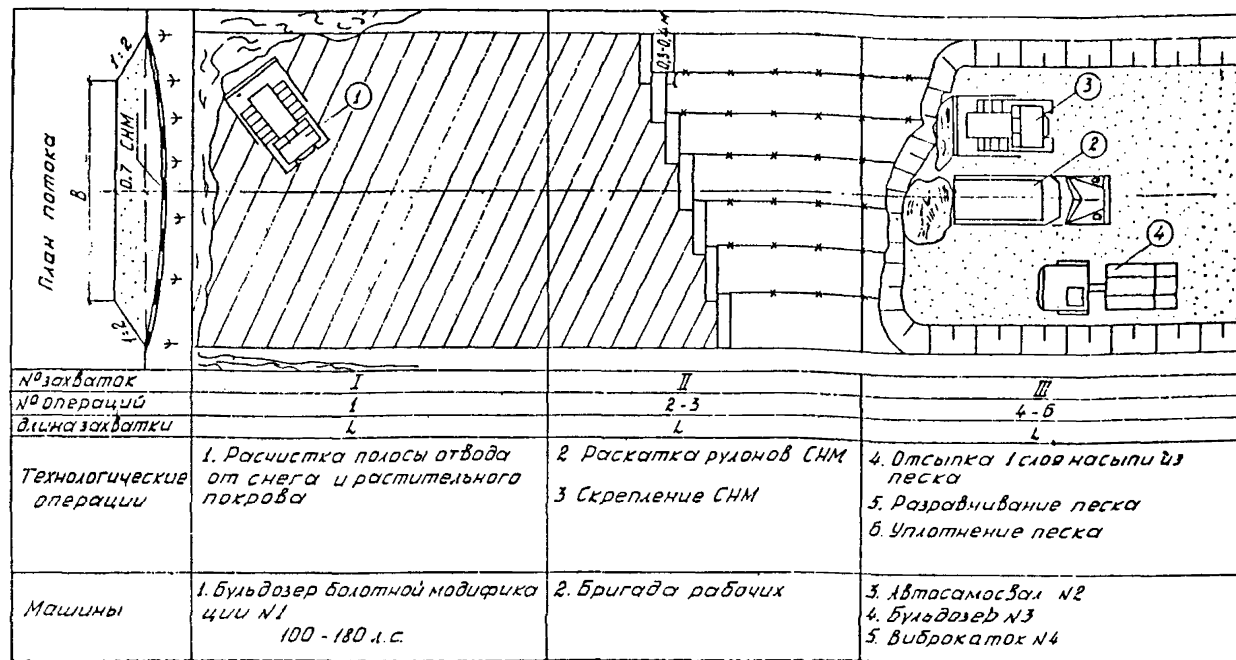
Рис. 24. Технологическая схема строительства автомобильной дороги с использованием СММ и торфа в нижней части насыпи (подготовительные работы и устройство торфяной части насыпи рекомендуется выполнять зимой). Условия применения: глубокие болота I типа и болота II типа при разработке торфа из боковых резервов
