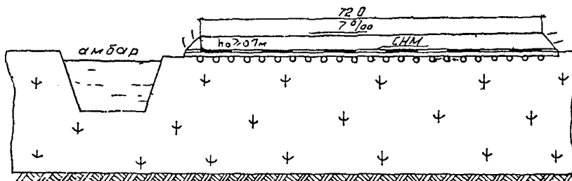
Рис. 12. Конструкция кустового основания на болотах I—III типов при расчетной толщине насыпного слоя более 1,5 м и отсыпке насыпи из однородных песков
