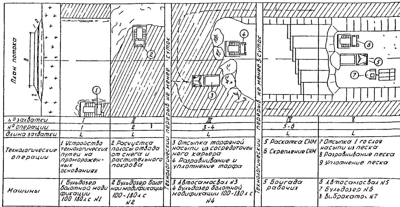
Рис. 25. Технологическая схема строительства автомобильной дороги и кустового основания с использованием СМ и торфяных грунтов в нижней части насыпи. Условия применения: болота I—III типов, вечномерзлые грунты с льдистостью от 0,25 до 0,40 при разработке из сосредоточенных резервов
