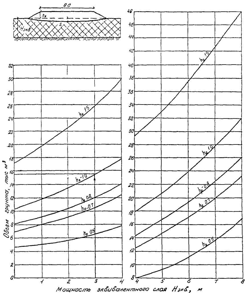
Рис. 30. График определения требуемого объема грунта для строительства 1 км дороги при ширине земляного полотна 8,0 м (насыпь на СНМ)
