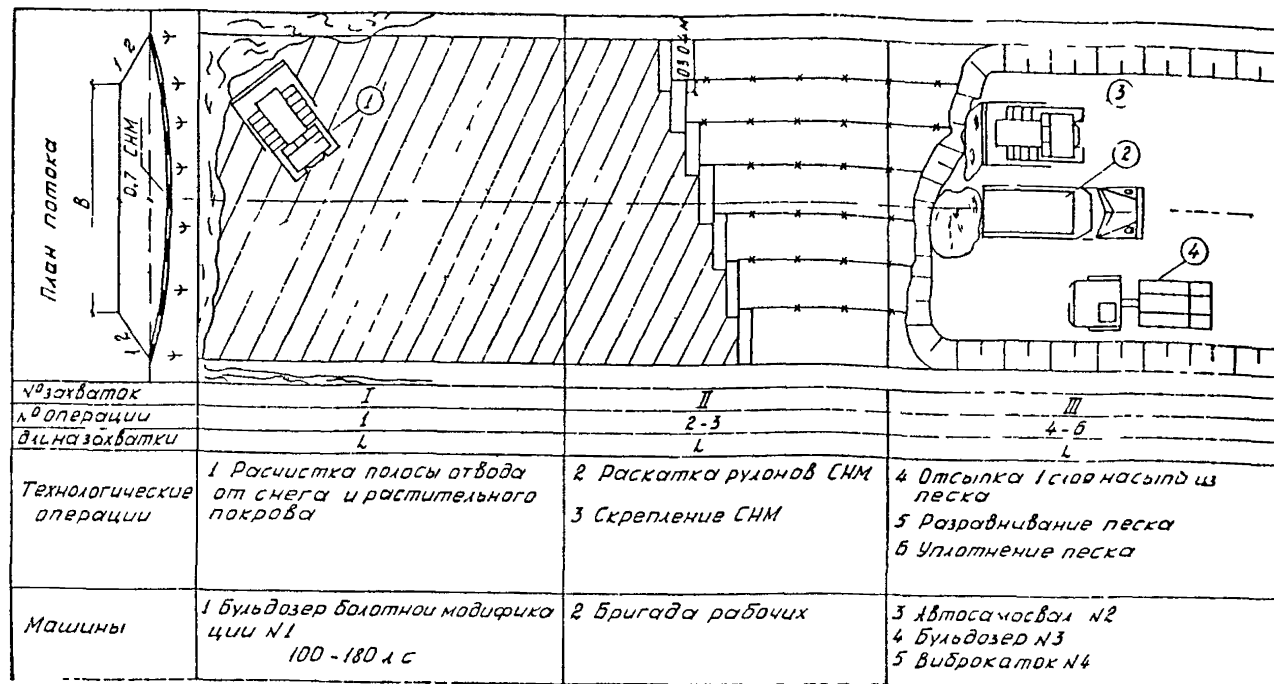
Рис. 22. Технологическая схема строительства автомобильной дороги и кустового основания с использованием СНМ в летний период (подготовительные работы рекомендуется выполнять зимой). Условия применения болота I и II типов, заторфованные грунты, вечномёрзлые торфяные грунты и минеральные грунты с льдистостью меньше 0,25
