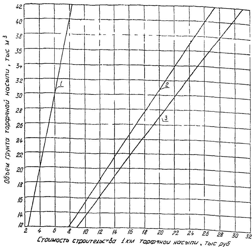
Рис. 29. График определения стоимости строительства 1 км торфяной насыпи в зависимости от способа разработки и дальности транспортирования торфа: 1 — торф из боковых резервов, 2 — торф из сосредоточенного резерва при дальности транспортирования 1 км, 3 — то же, при дальности транспортирования 2 км
