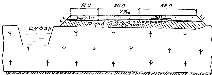
Рис. 10. Конструкция оснований под куст скважин на вечномёрзлых грунтах с просадочностью в пределах 0,03—0,15 и болотах II, III типов
