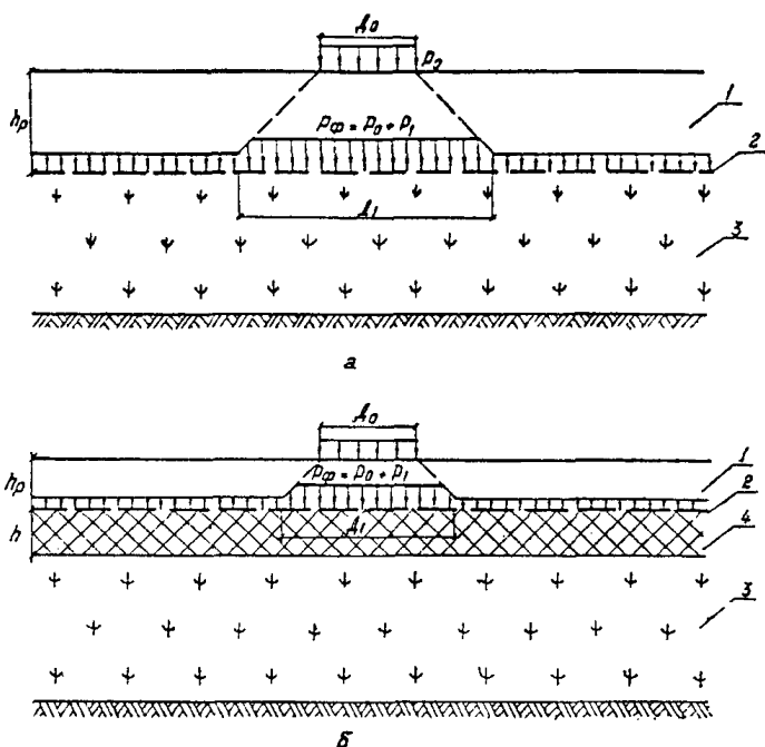
Рис. 20. Расчетная схема для определения толщины насыпного слоя: а — конструкция по типу 1; б — конструкция по типу 2; 1 — насыпной грунт; 2 — текстильная прослойка; 3 — слабое основание; 4 — насыпной торф
