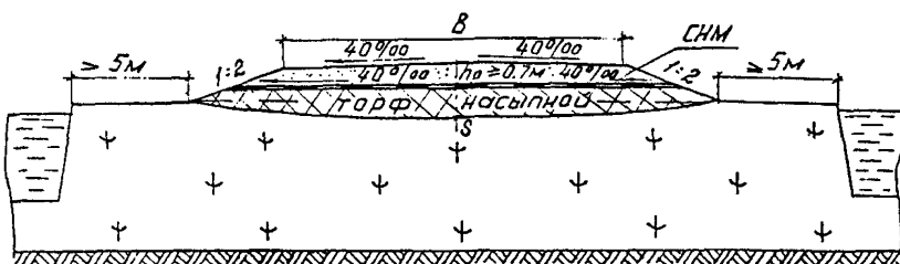
Рис. 9. Конструкция автомобильной дороги на глубоких болотах I типа и болотах II типа при отсыпке торфяной части насыпи из боковых резервов
