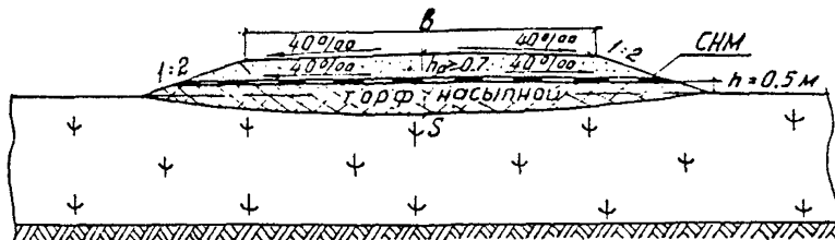
Рис. 8. Конструкция автомобильной дороги на вечномёрзлых грунтах с просадочностью в пределах 0,03—0,15 и на болотах II, III типов при отсыпке торфяной части насыпи из сосредоточенных карьеров
