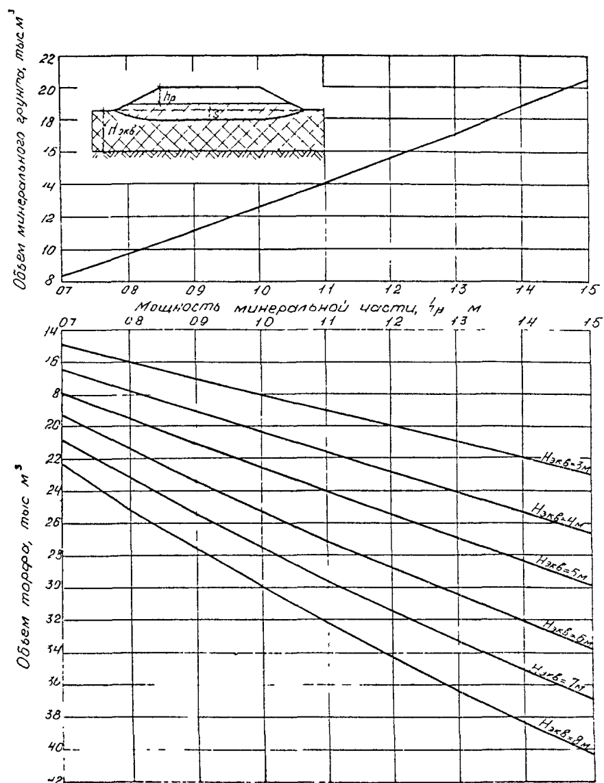
Рис. 33. График определения требуемых объемов грунтов (песка и торфа) для строительства 1 км дороги при ширине земляного полотна 10 м
