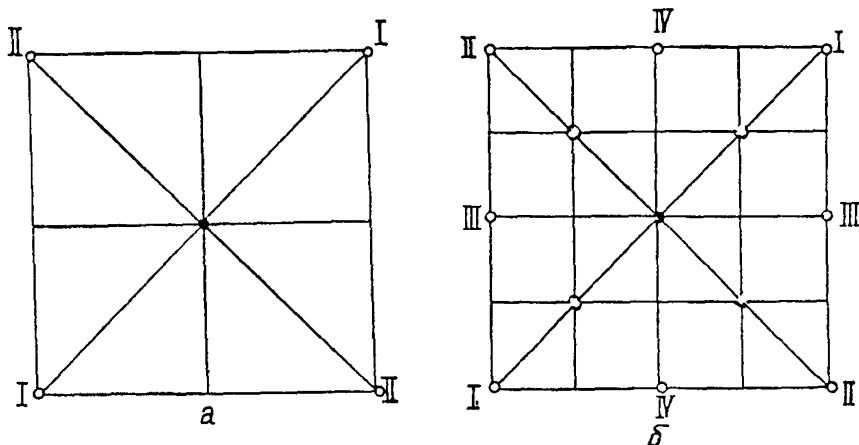
Рис. 4. Схема расположения скважин на площадке под кустовое основание: а — при однородных по глубине и простиранию грунта; б — при неоднородных грунтовых условиях; ● — опорная скважина; ○ — зондировочная скважина; I—I — линия построения инженерно-геологического разреза
