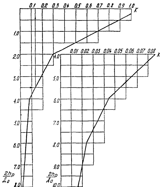
Рис. 19. Номограмма для определения коэффициента распределения напряжений в зависимости от 2h_p/D_0 : а — от 0 до 8,0; б — от 4,0 до 10,0
