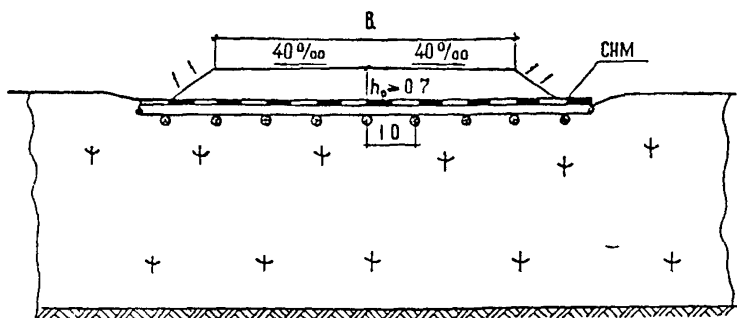
Рис. 13. Конструкция автомобильной дороги на болотах III типа при использовании древесины (слани) и СНМ в основании насыпи
