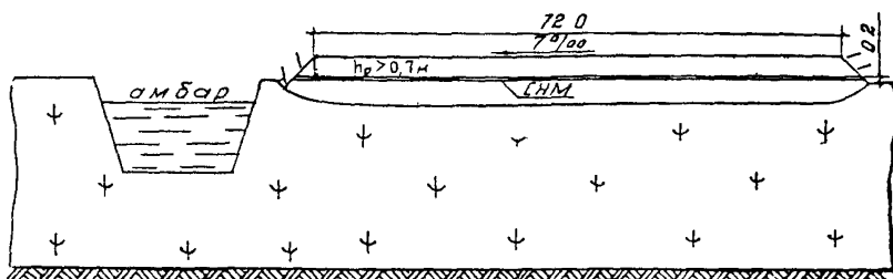
Рис. 14. Конструкция кустового основания на болотах III типа при использовании древесины (слани) и СНМ в основании насыпи
