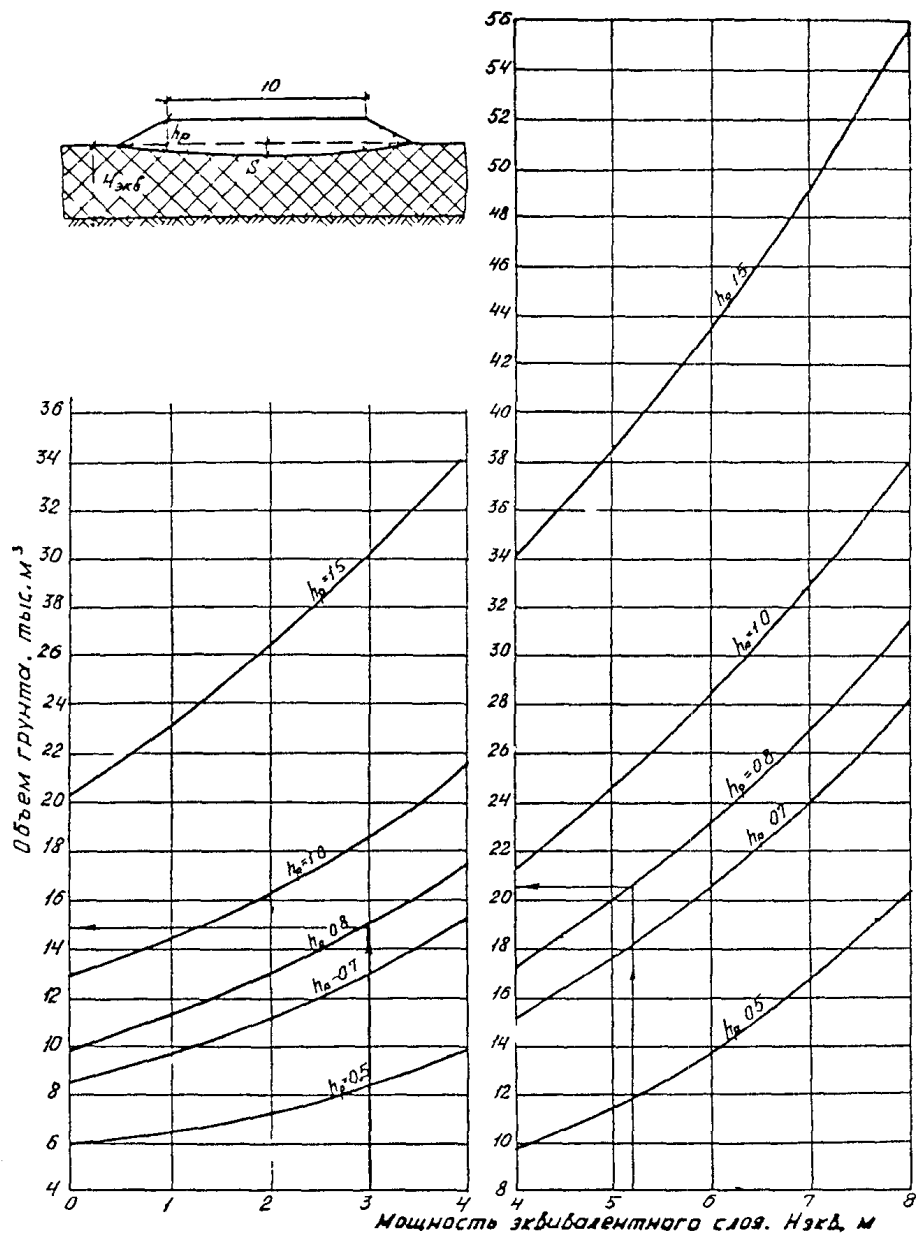
Рис. 31. График определения требуемого объема грунта для строительства 1 км дороги при ширине земляного полотна 10 м (насыпь на СНМ)
