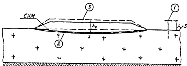
Рис. 21. Схема отсыпки насыпи на СНМ: 1 — высотник, устанавливаемый на высоту h_p + S ; 2 — контур земляного полотна после консолидации основания; 3 — контур земляного полотна на момент отсыпки
