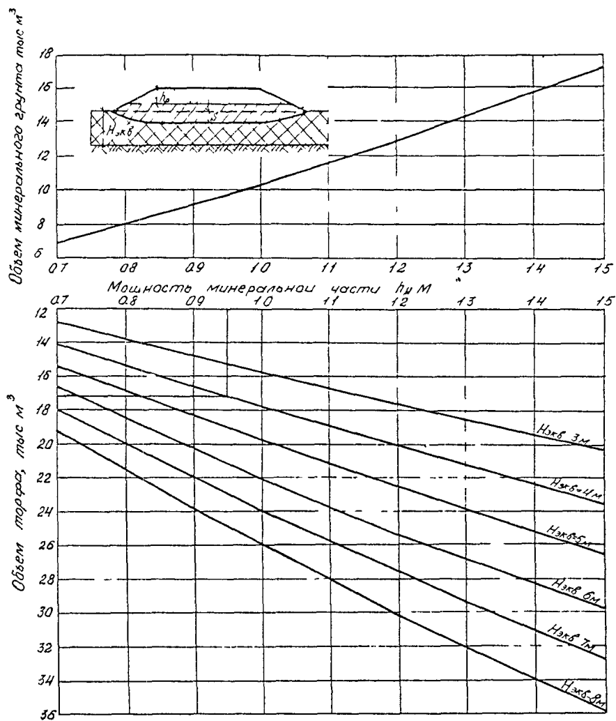
Рис 32 График определения требуемых объемов грунтов (песка и торфа) для строительства 1 км дороги при ширине земляного полотна 8 м
