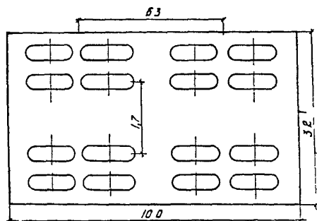
Рис. 1. Размеры и схема расстановки колес (от самолета ТУ-104) тележки для перевозки бурового оборудования (вес тележки — 15 тс; грузоподъемность — 100 тс)
