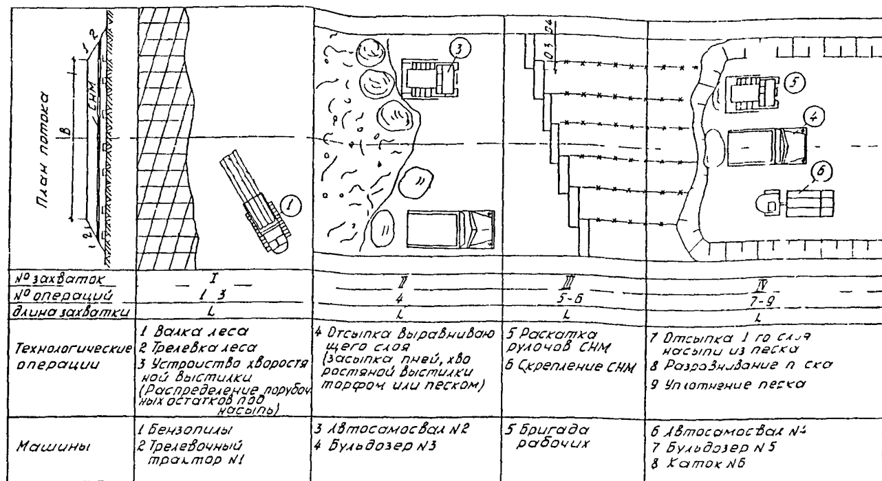
Рис. 23. Технологическая схема строительства автомобильной дороги с использованием СМ на переувлажненных минеральных грунтах
