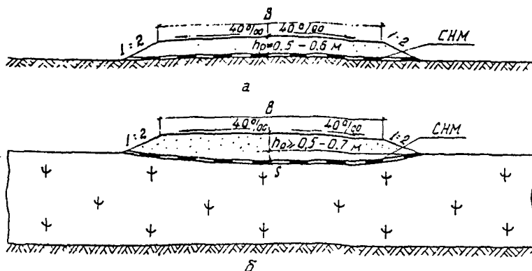
Рис. 6. Конструкция автомобильной дороги: а — на минеральных и вечномерзлых грунтах с просадочностью \delta_{\text{п}} менее 0,03; б — на болотах I, II типов и заторфованных грунтах
