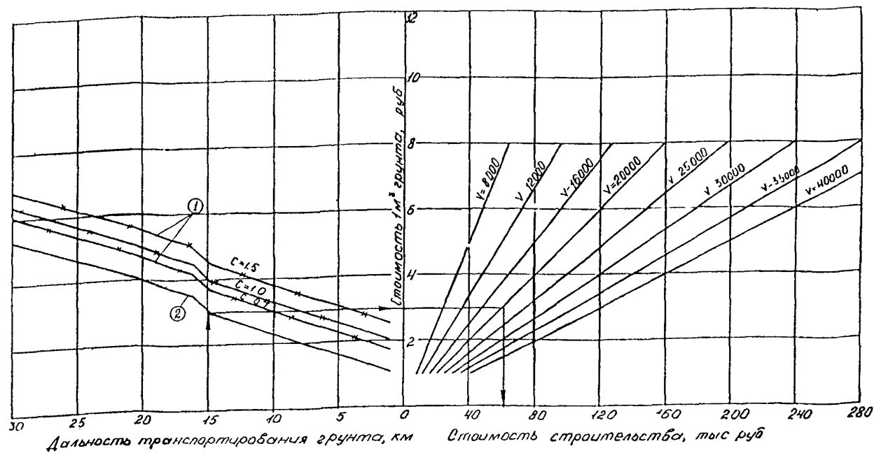
Рис. 28. График определения стоимости строительства земляного полотна в зависимости от дальности транспортирования, способа разработки и объема грунта, укладываемого в насыпь: 1 — грунт из сосредоточенного карьера; 2 — грунт гидронамывной
