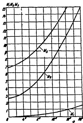
Рис 18. Номограмма для определения функций в зависимости от угла внутреннего трения слабого грунта
