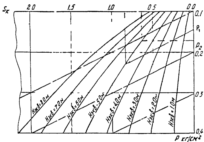
Рис. 16. Номограмма для определения величин конечных осадок (сплошная стрелка показывает последовательность определения осадок для песчаной насыпи, пунктирная — для конструкции с торфом в нижней части; \gamma_{об} песка 1,8 г/см 3 )
