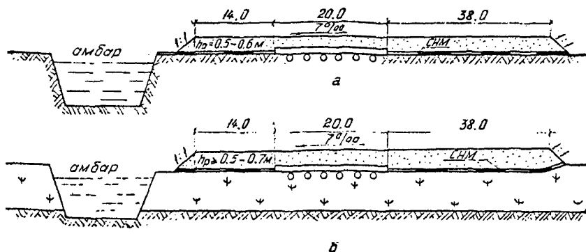
Рис. 7. Конструкция основания под куст свай: а — на минеральных и вечномерзлых грунтах с просадочностью \delta_{\text{п}} менее 0,03; б — на болотах I, II типов и заторфованных грунтах
