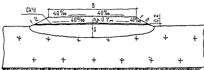
Рис. 11. Конструкция автомобильной дороги на болотах I—III типов при расчетной толщине насыпного слоя более 1,5 м и отсыпке насыпи из однородных песков
