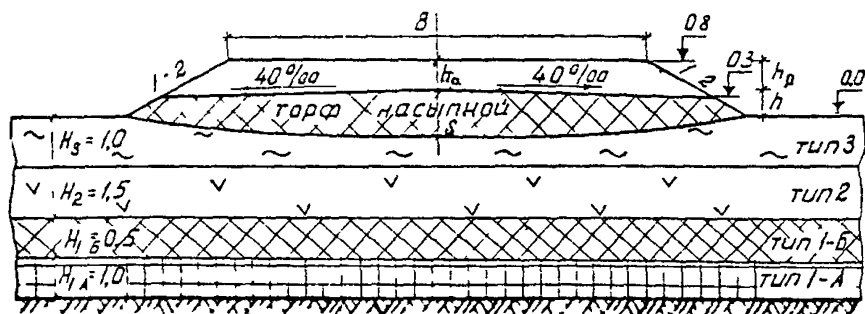
Рис. 15. Расчетная схема определения на болотах величин конечных осадок
