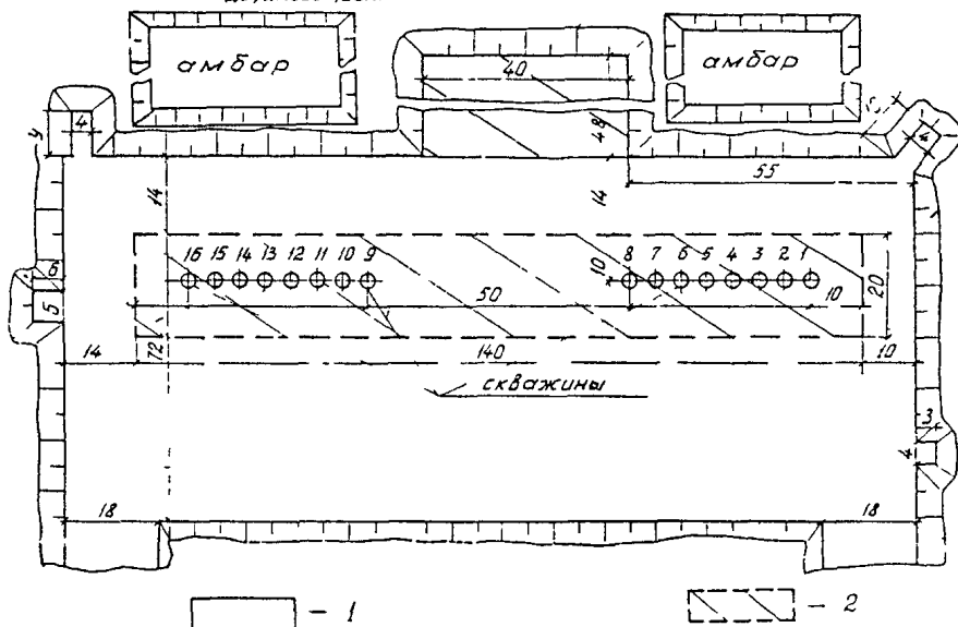
Рис. 2. План основания под кусты скважин, размеры даны в метрах (трубопроводы на слабых грунтах укладываются на сплошной деревянный настил): 1 — возможная площадь укладки СНМ; 2 — обязательная площадь укладки древесины
