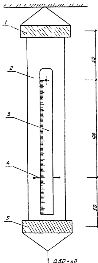
Рис. 27 Схема испытания СММ на растяжение и разрывную нагрузку 1 — верхний зажим, 2 — синтетический нетканый материал, 3 — линейка, 4 — металлическая шпилька, 5 — нижний зажим
