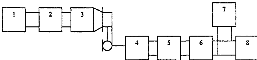
1 - селективный вольтметр; 2 - усилительно-питающее устройство; 3 - искусственное ухо, 4 - испытуемый ЦТА; 5 - блок сопряжения; 6 - эталонный кодек; 7 - электронный вольтметр; 8 - генератор сигналов низкочастотный.
