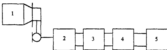
1 - искусственное ухо; 2 - испытуемый ЦТА, 3 – блок сопряжения; 4 - эталонный кодек; 5 – психометр.
