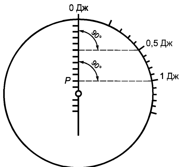
Рисунок 1.7 — Градуировка шкалы
