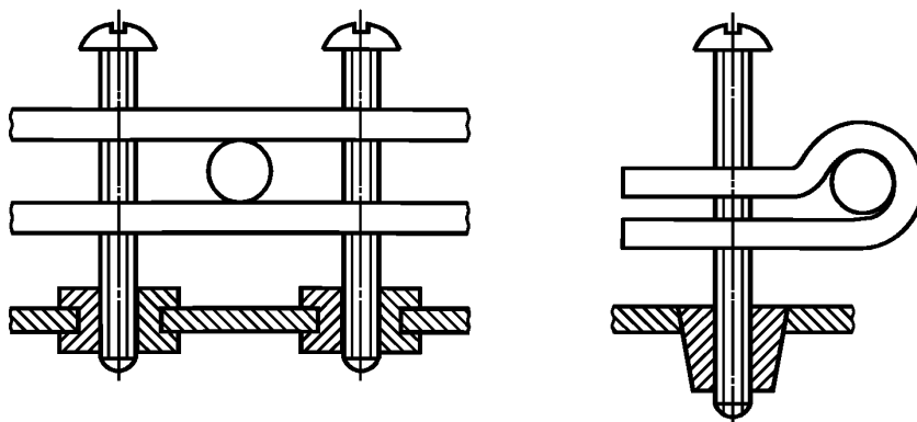
б) Недопустимые конструкции
