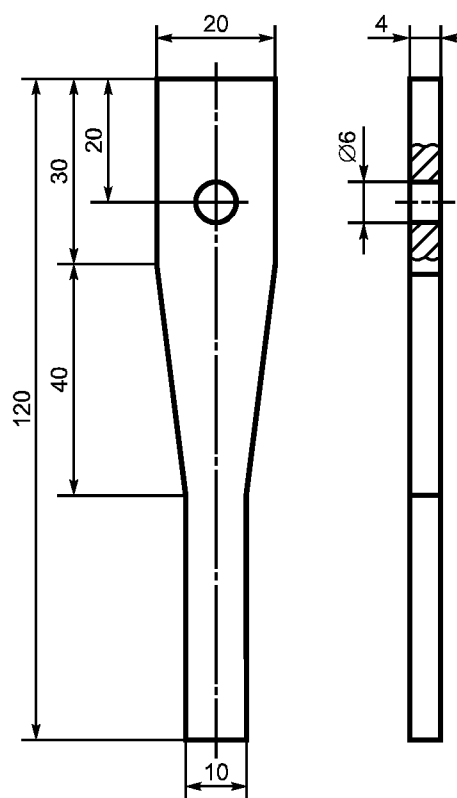
Рисунок 1.3 — Стальная пружина
