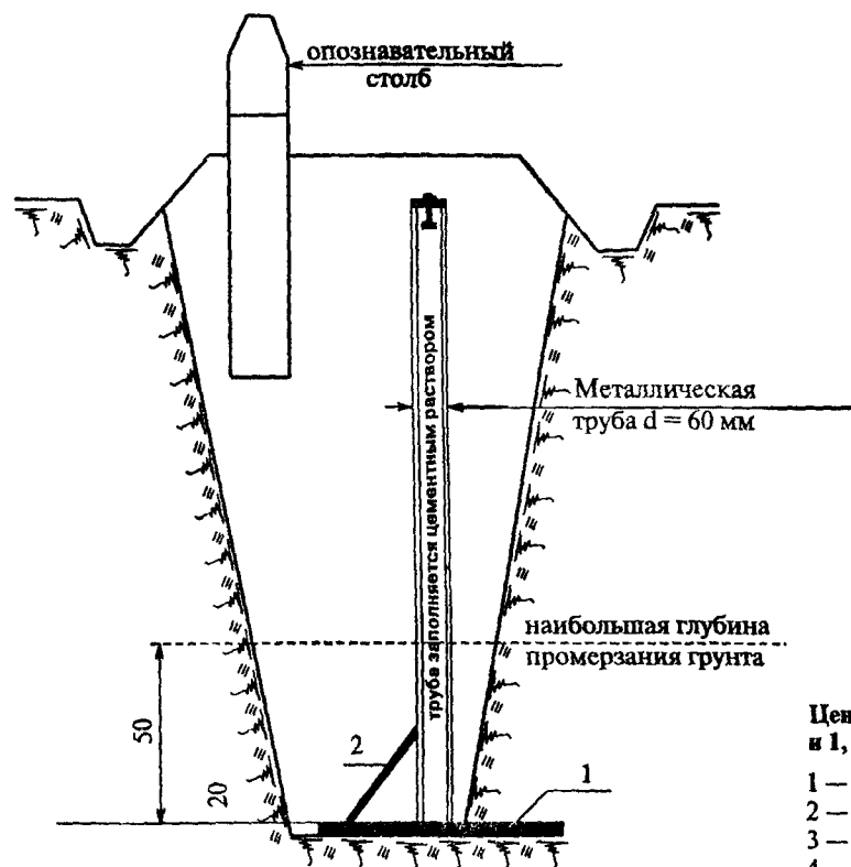
Центр пункта триангуляции, полигонометрии 4 кл. и 1, 2 разрядов, грунтовой репер нивелирной сети III–IV кл. для труднодоступных районов 1 — стальная пластина 50 x 50 см, толщиной 5–10 мм, приваренная к трубе 2 — арматурное крепление
