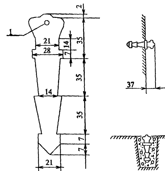
Стенной знак пункта полигонометрии 4 кл. и 1, 2 разрядов
