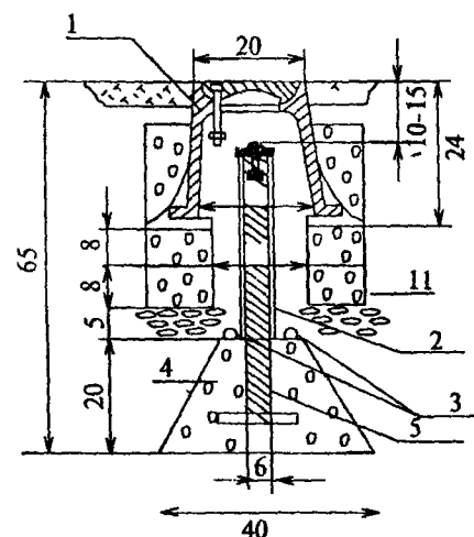
Центр пункта триангуляции, полигонометрии 4 кл. и 1, 2 разрядов, в районах сезонного промерзания грунта
