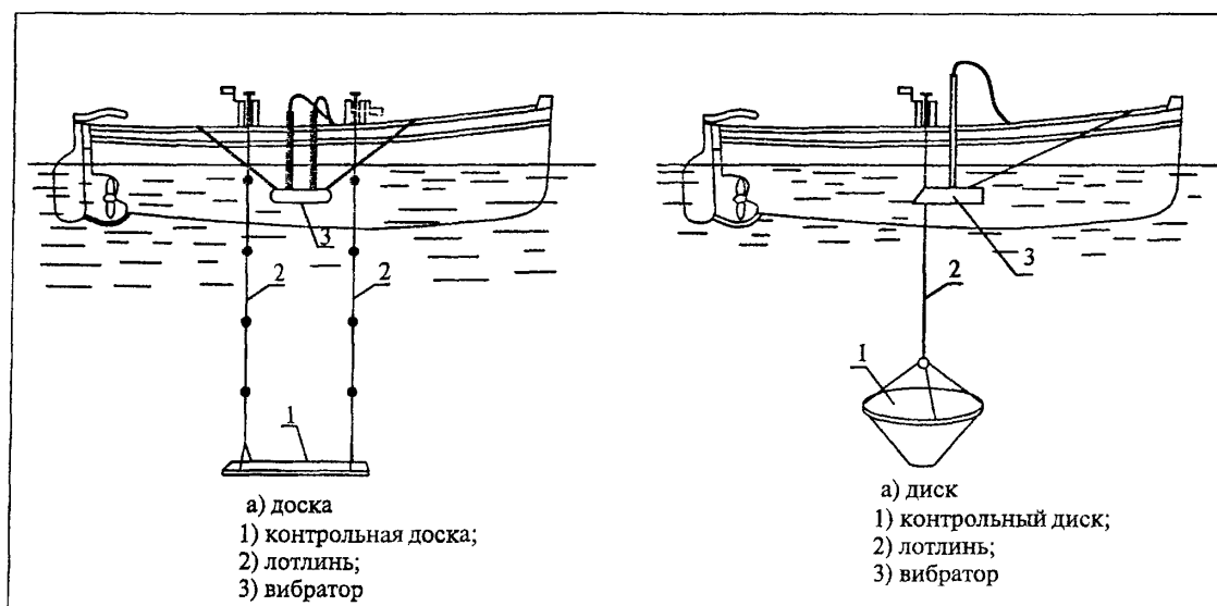
Рис. 3. Тарирующие устройства эхолота.
