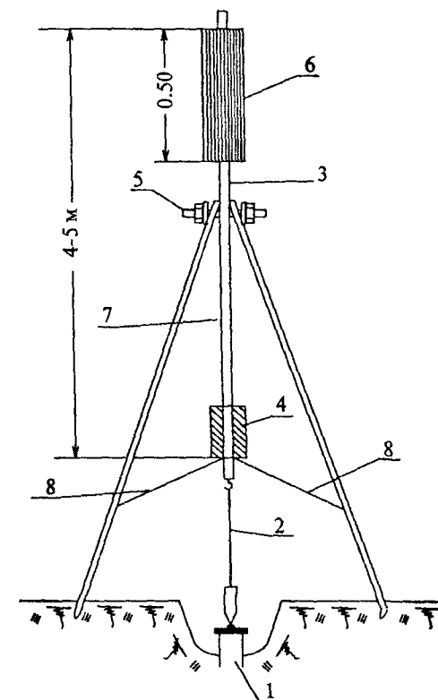
Металлическая или деревянная веха с противовесом
