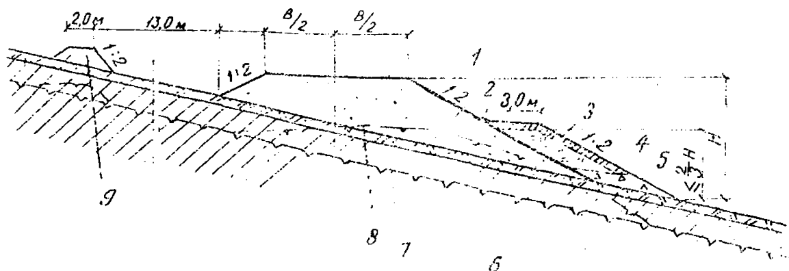
Рис. 3. Поперечный профиль насыпи на косогорных участках местности, сложенных вечномёрзлыми минеральными грунтами: 1 — вёсок крупно- или среднезернистый или легкий суглинок; 2 — мохорастительный покров; 3 — берма из торфа; 4 — защитный слой из глины толщиной 0,2 м; 5 — дренаж из крупнозернистого песка или гравия; 6 — грунт основания с W_c > 0,8 < W_{тет} ; 7 — ВГВМГ до постройки насыпи; 8 — ВГВМГ после постройки насыпи; 9 — мерзлотный валик из глинистого грунта.
