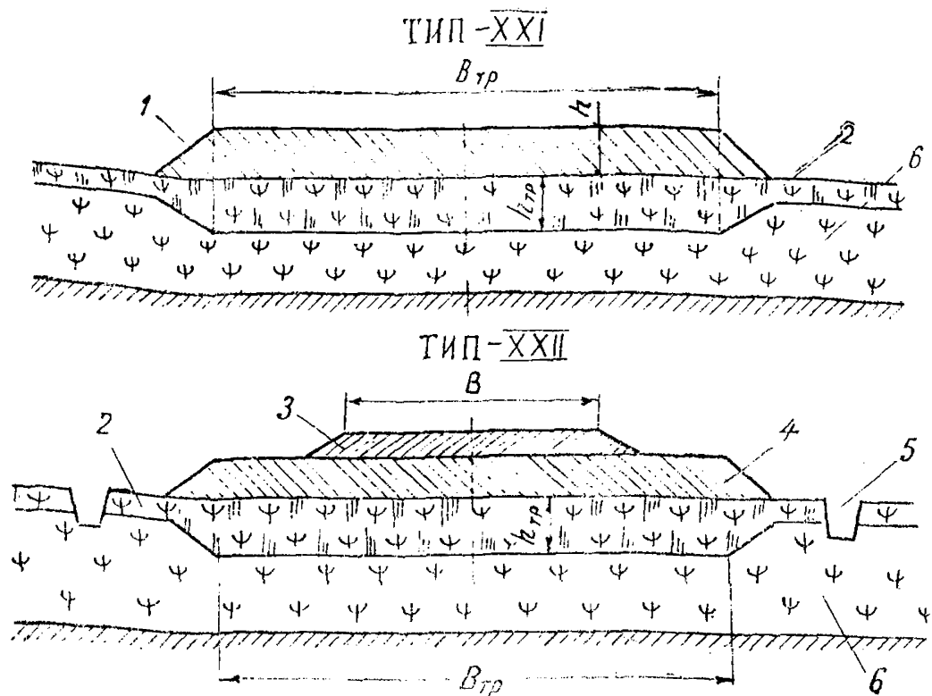
Рис. 27. Поперечные профили автозимников с продленными сроками эксплуатации на болотах: 1 — дорожное покрытие из снегольда или смеси снегольда с добавками (моховой очес, древесные опилки, щепа, стружка); 2 — замороженное торфяное основание; 3 — земляное полотно; 4 — теплоизолирующее полотно из смеси снега с моховым очесом; 5 — боковые водоводные каналы; 6 — талый слой болота.
