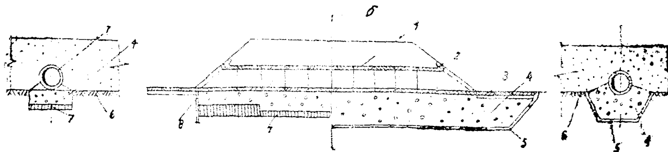
Рис. 14. Конструкция труб на местности без вечномерзлых грунтов с устройством теплоизолирующего слоя в основании (а) или капилляропрерывающей прослойки (б): 1 — тело трубы; 2 — воротниковый оголовок; 3 — отсыпка; 4 — грунт замены; 5 — капилляро прерывающий слой; 6 — пучинистый грунт; 7 — теплоизолирующий слой; 8 — глиняный экран.
