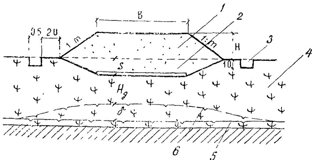
Рис. 7. Поперечный профиль насыпи на заторфованных болотах: 1 — песок; 2 — сланевый настил из бревен \varnothing 15 см; 3 — осадочные прорези; 4 — горф устойчивой консолидации; 5 — ВГВМГ до постройки насыпи, 6 — ВГВМГ после постройки насыпи.
