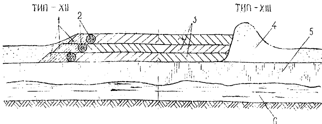
Рис. 22. Усиление ледяного покрова методом послойного намораживания льда: 1 — пригравированный снег; 2 — жерди; 3 — намораживаемые слои; 4 — валик из снега; 5 — естественный ледяной покров; 6 — вода.
