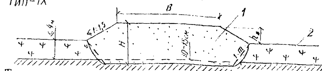
Тип-X
