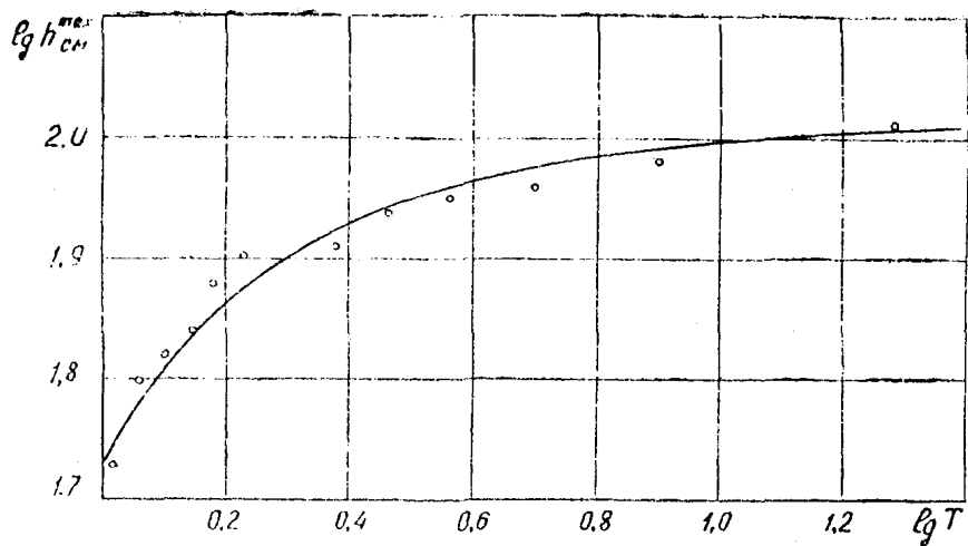
Рис. 1. График для определения величины HP_{сн} (для ст. Надым).
