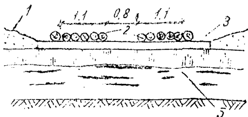
Тип XIV
