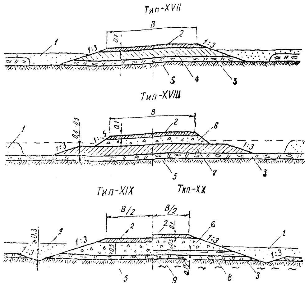
Рис. 26. Поперечные профили автозимников с продленными сроками эксплуатации: 1 — снеговой покров; 2 — уплотненный слой снега на полотне дороги; 3 — естественный мохорастительный покров; 4 — теплоизолирующее полотно из смеси снега со мхом; 5 — мерзлое грунтовое основание; 6 — земляное полотно; 7 — полотно из уплотненного снега; 8 — хворостяная выстилка или сплошной настил из тонкомерной древесины; 9 — сильнольдистый грунт основания.
