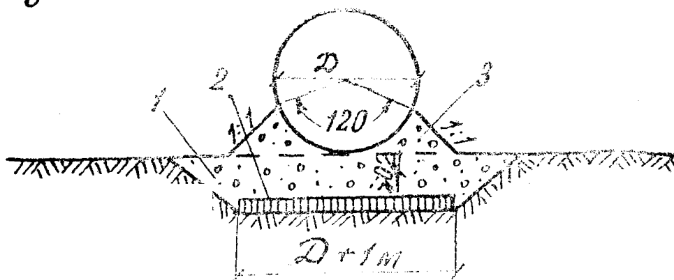
Рис. 32. Типы оснований под гофрированные трубы: а—при укладке на спрофилированное ложе; б—при укладке на горизонтальную поверхность подушки; 1—грунт подушки; 2—теплоизоляционный слой из пенопласта или мохоторфа; 3—грунт подбивки.
