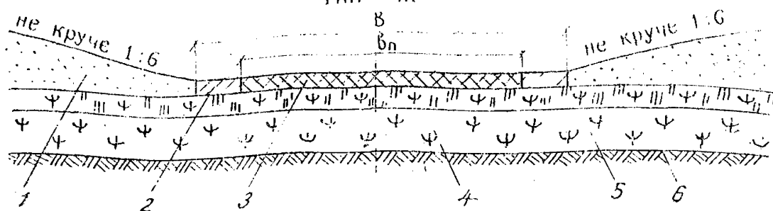
ТИП - IX
