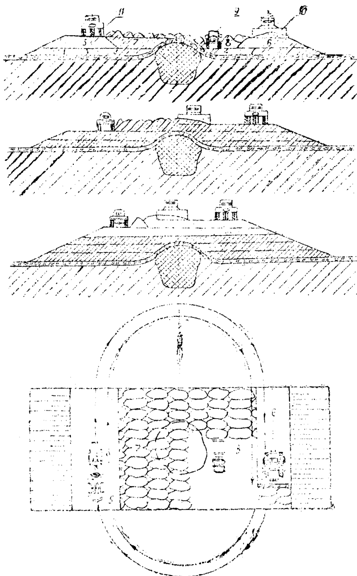
Рис. 1. Возведение насыпи из глинистого грунта на мелких буграх пучения (первый принцип проектирования): 1—8—последовательность отсыпки грунта; 9—автомобиль КРАЗ-256Б; 10—бульдозер ДЗ-54С; 11—каток ДУ-39А.
