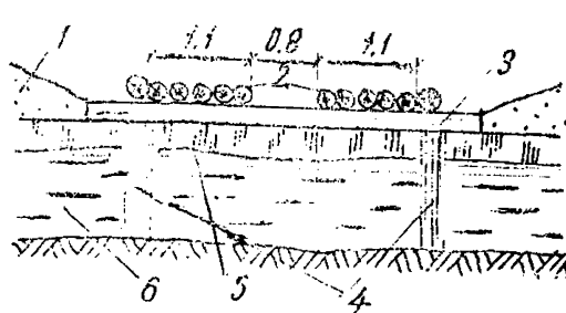
Рис. 23. Усиление ледяных переправ деревянным настилом: 1 — снеговой покров; 2 — колесопроводы; 3 — поперечины; 4 — стойки; 5 — естественный ледяной покров; 6 — вода.
