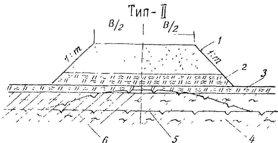
Рис. 2 Поперечный профиль насыпи на льдистом минеральном грунте (пылеватый суглинок) 1 — крупно- или среднезернистый песок; 2 — теплоизолирующий слой из торфа; 3 — мохогорфяной слой; 4 — пылеватый суглинок льдистый; 5 — ВГВМГ до постройки насыпи; 6 — ВГВМГ после постройки насыпи.
