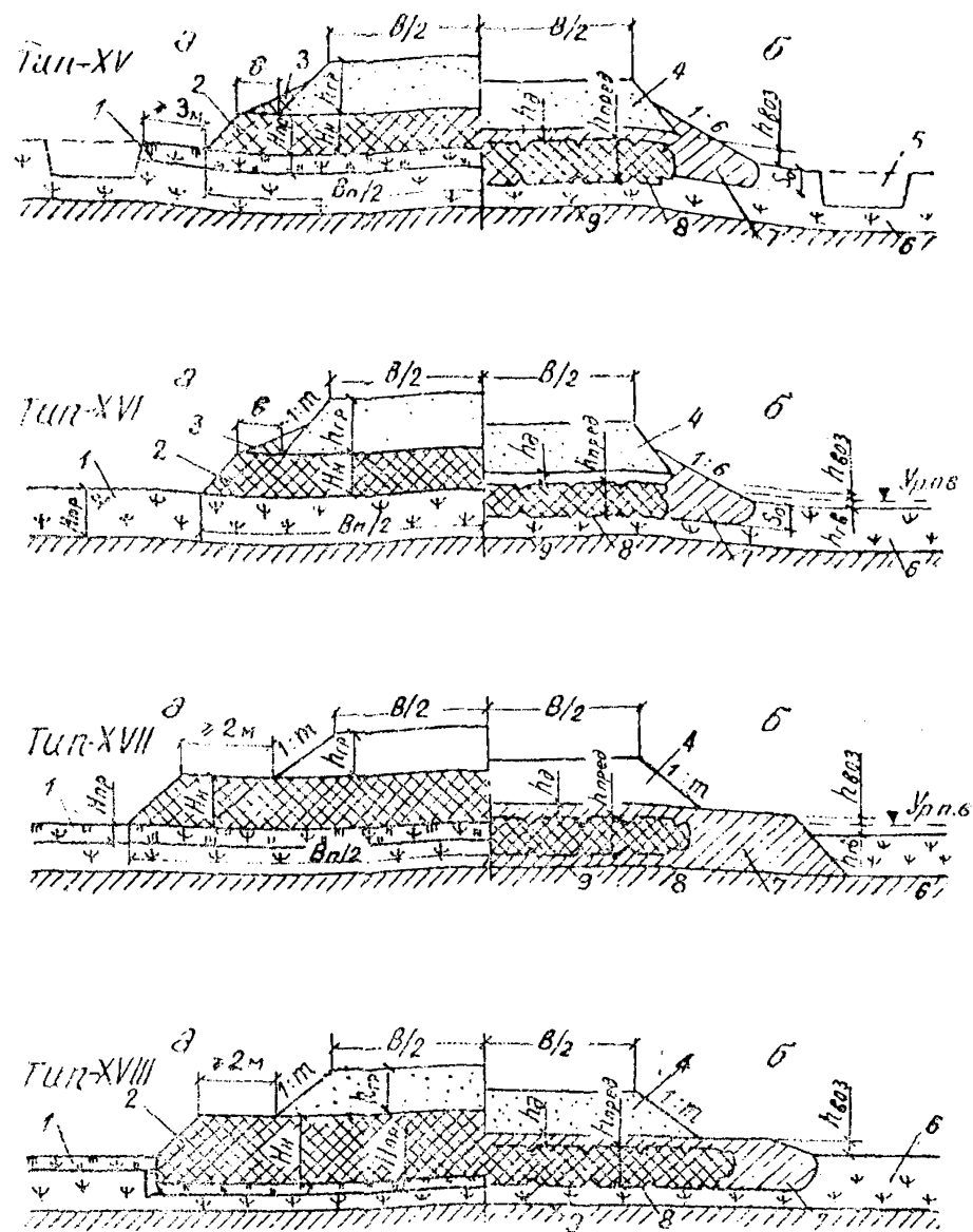
Рис. 10. Поперечные профили насыпей на промороженных основаниях в период строительства (а) и в процессе эксплуатации на конец теплого периода года (б): 1 — промороженный слой естественной торфяной залежи; 2 — намороженная торфяная плита; 3 — боковые призмы из торфа; 4 — насыпь из минерального грунта; 5 — боковой резерв; 6 — талый слой торфяной залежи; 7 — талые слои торфяной плиты; 8 — граница мерзлого торфяного основания; 9 — минеральное дно болота.
