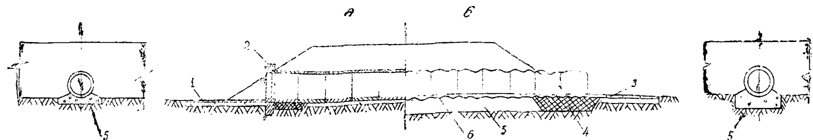
Рис. 12. Конструкции бесфундаментных водопропускных железобетонных (а) и металлических гофрированных (б) труб: 1 — отмостка из местного материала; 2 — порталный оголовок; 3 — отмостка из бетонных плит; 4 — теплоизолирующий слой; 5 — выравнивающий слой из песчано-гравийного материала; 6 — битумная отмостка.
