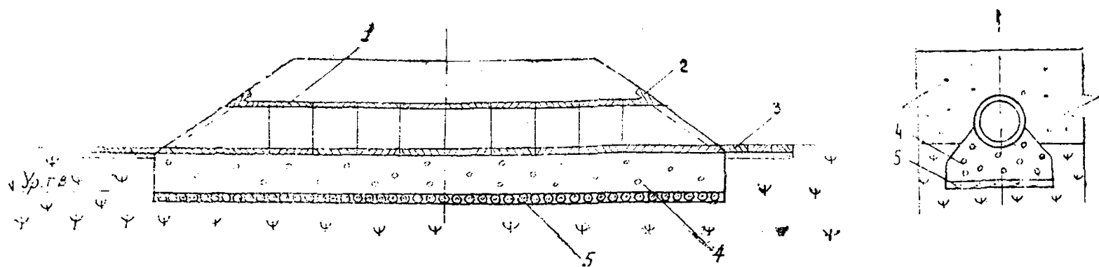
Рис. 13. Конструкция бесфундаментной трубы на сланевом настиле: 1 — тело трубы; 2 — воротниковый оголовок; 3 — отмостка из бетонных плит; 4 — грунт замены; 5 — сланевый настил.
