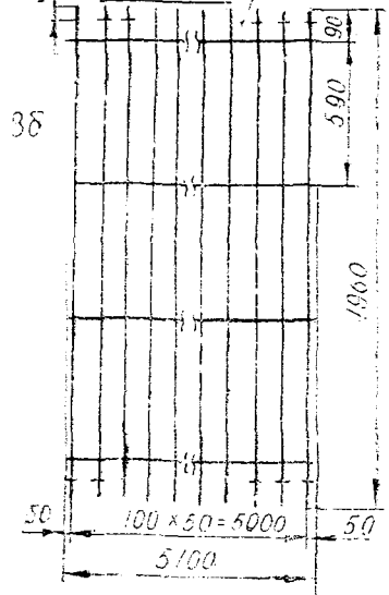
Сетка С4
