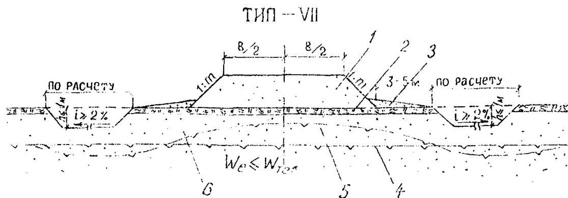
Рис. 6. Поперечный профиль насыпи на сухих водораздельных участках со сливающейся вечной мерзлотой: 1 — средне- или крупнозернистый песок; 2 — мохорастительный покров; 3 — берма; 4 — ВГВМГ до постройки насыпи; 5 — ВГВМГ после постройки насыпи; 6 — мелко- или среднезернистый песок; супесь.
