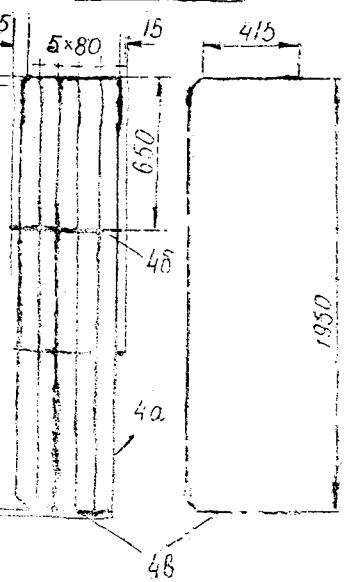
Сетка С5
