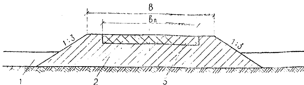
ТИП - X
