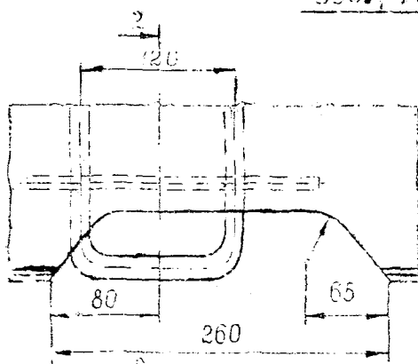
Сетка С4
