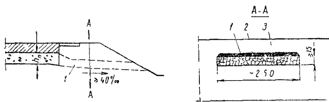
Рис. 7. Уширенный поперечный дренаж h_{II} — толщина дренирующего слоя, 1 — дренажная воронка, заполненная щебнем или гравием; 2 — толь или рубероид, 3 — местный грунт
