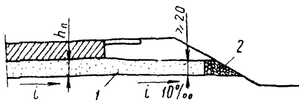
Рис. 9. Сплошной дренирующий слой под обочинами:
