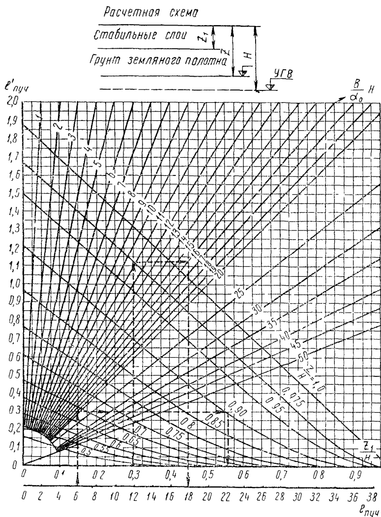
Рис. 15 Номограмма для расчета конструкций на морозоустойчивость
