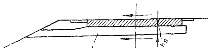
Рис. 6. Дренажный слой при односкатном поперечном профиле проезжей части.
