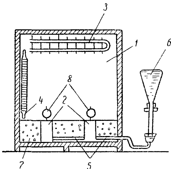
Рис. 3. Схема холодильной установки:
