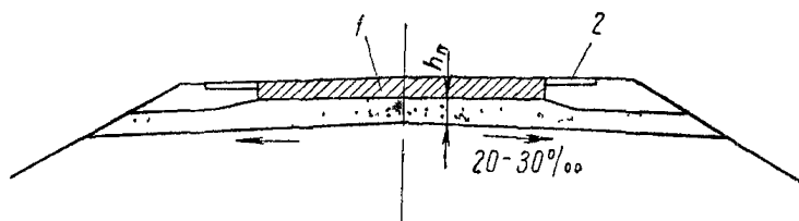
Рис. 5. Дренажный слой при двухскатном поперечном профиле проезжей части
