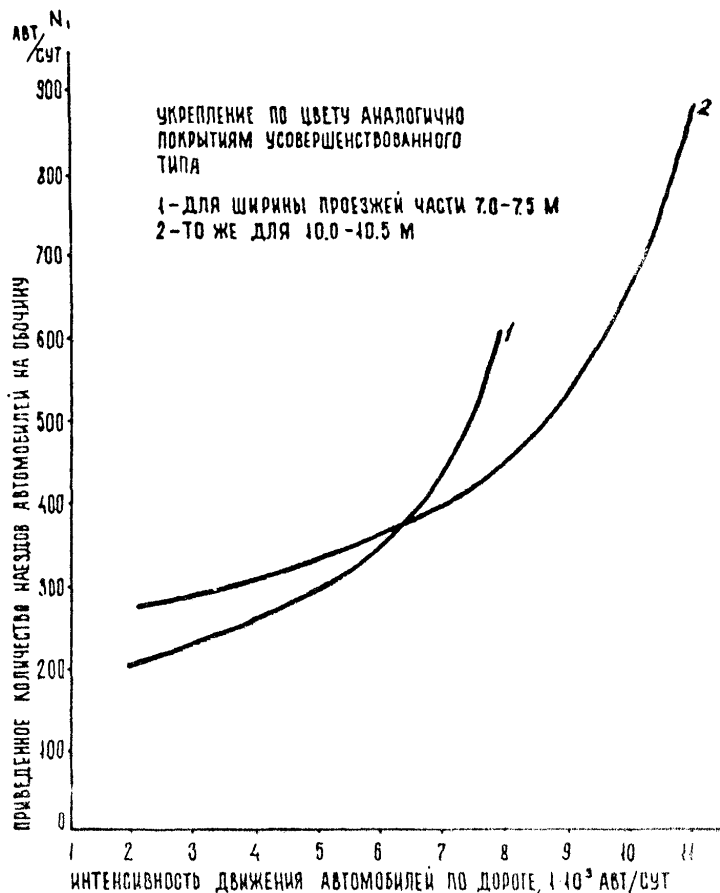
Рис. I. График расчетных значений количества наездов автомобилей на обочину в зависимости от интенсивности движения при цвете верхнего слоя укрепления обочин аналогичном покрытиям усовершенствованного типа
