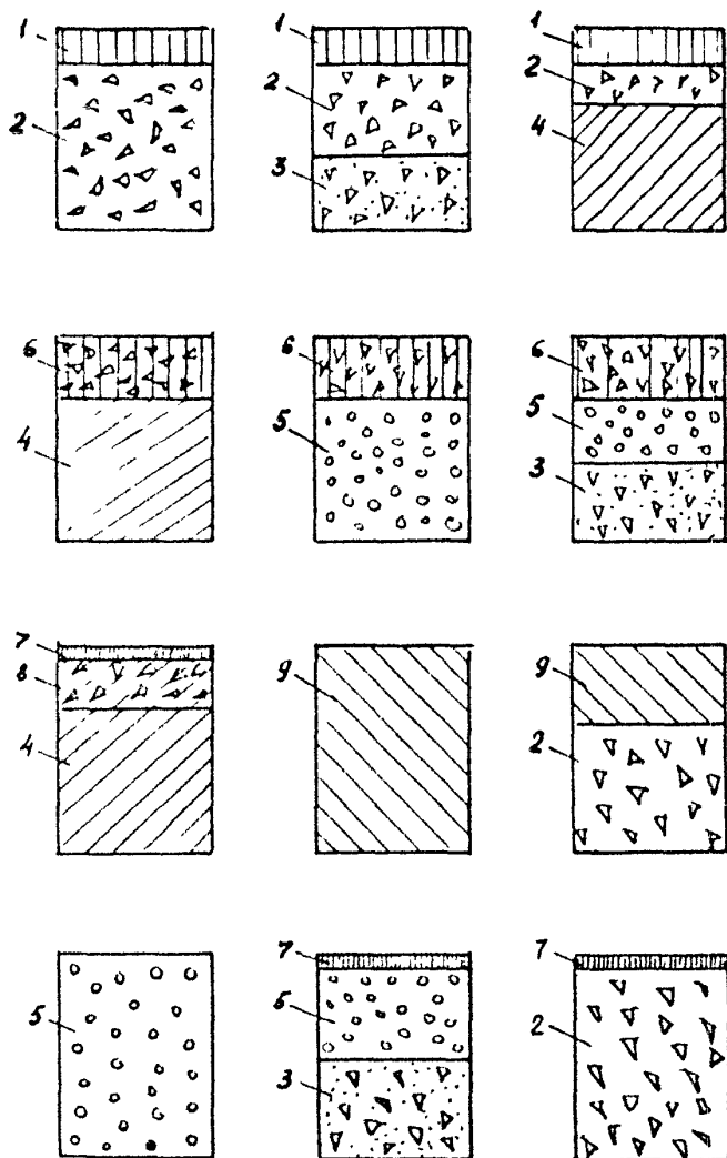
Рис. 5. Конструкция укрепления обочины
