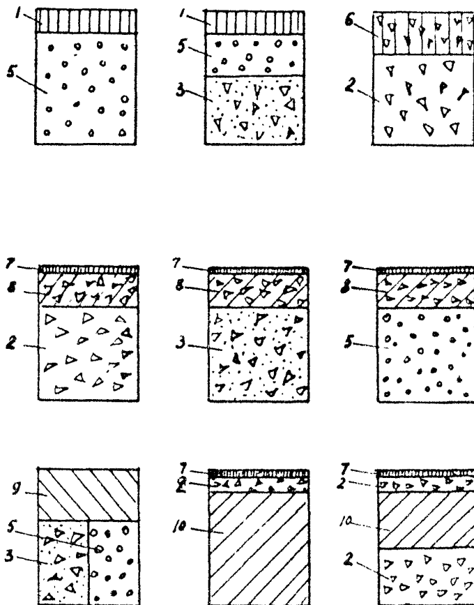
Рис. 5. Конструкции укрепления забочин
