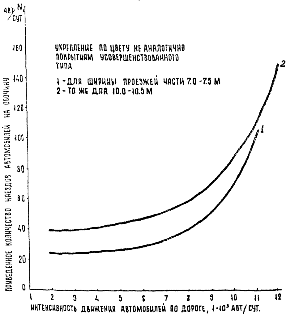
Рис. 2. График расчетных значений количества наездов автомобилей на обочину в зависимости от интенсивности движения при цвете верхнего слоя обочины, не аналогичном покрытиям усовершенствованного типа
