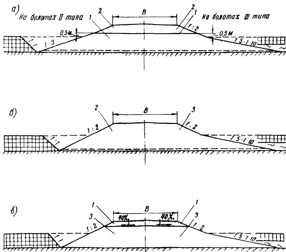
Рис.2. Конструкция земельного полотна с полным выторфовыванием на болотах II и III типов:
