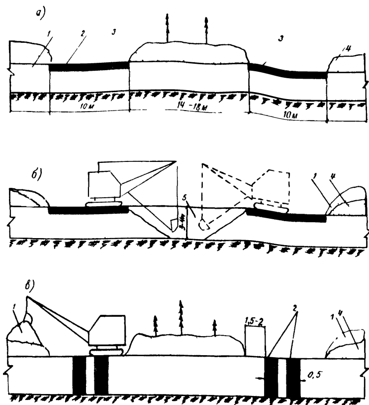
Рис.4. Проведение работ по выторфовыванию в зимний период:
