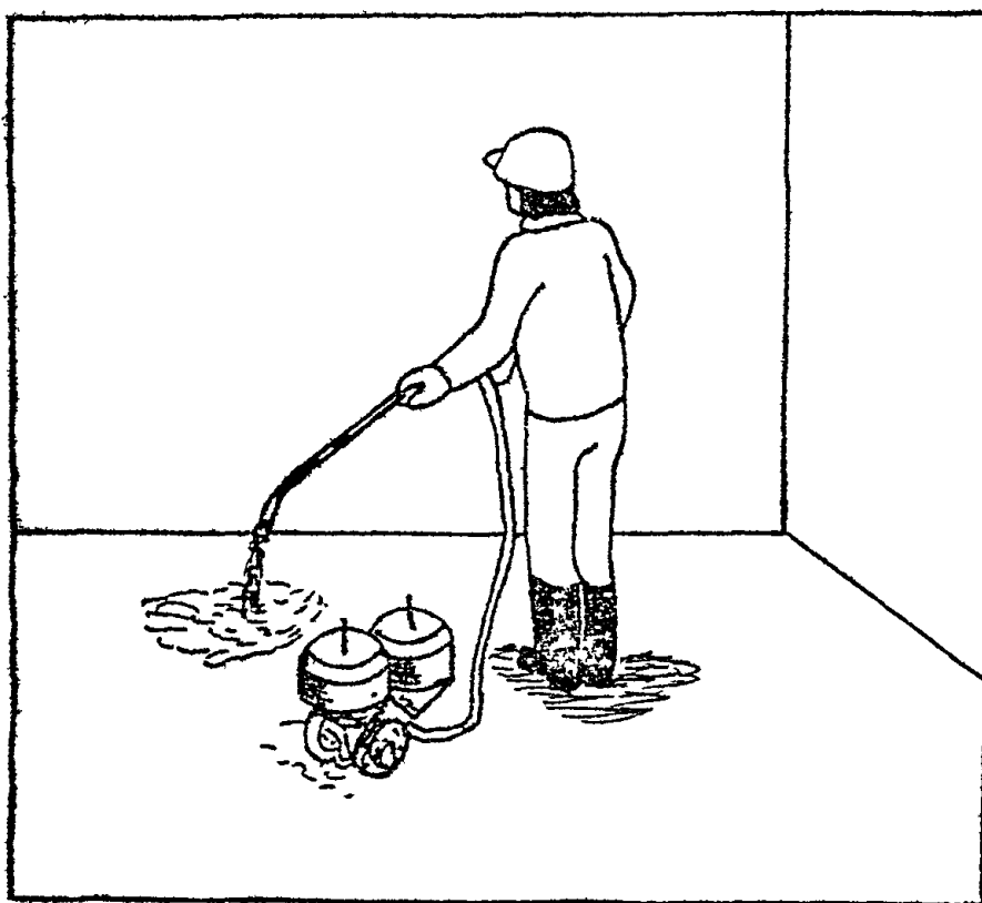
Рис. 2. Огрунтовка основания
