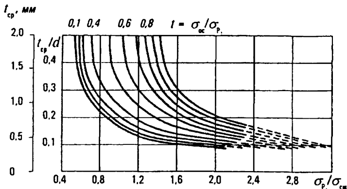
Рис. 6. Зависимости параметров дискования керна t_{cp}/d_{\text{дис}} от уровня напряженности массива \sigma_p/\sigma_{сж} при различных соотношениях между осевыми и радиальными напряжениями \sigma_{ос}/\sigma_p ; d_{\text{дис}} — диаметр дисков; t_{cp} — средняя толщина дисков.
