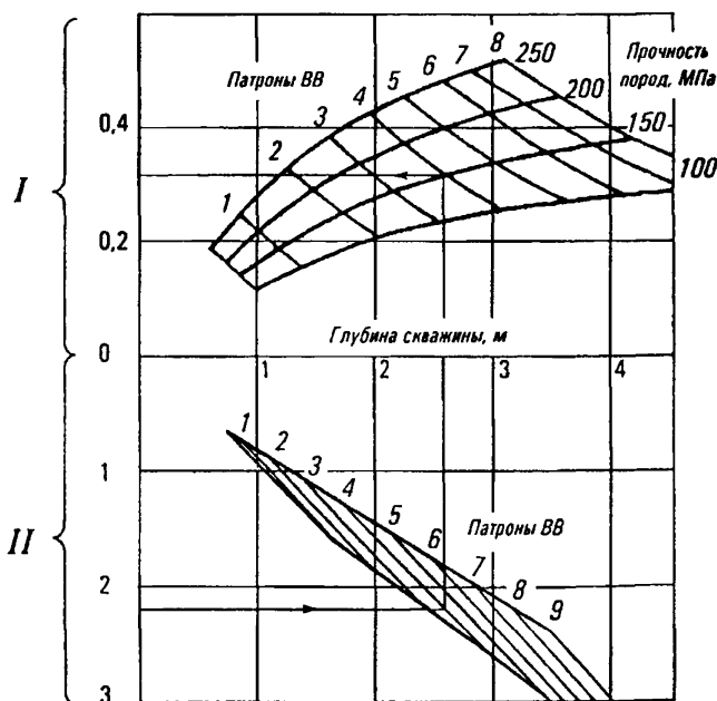
Рис. 2. Номограмма для определения параметров камуфлетного взрыва ряда шпуров (масса патронов ВВ 0,2 кг):
