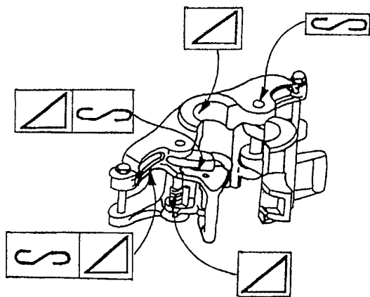
Рис. 5.8. Элеватор
