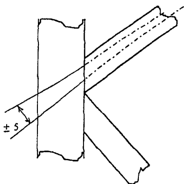
Рис. 2. Смещение осевой линии решетчатой конструкции
