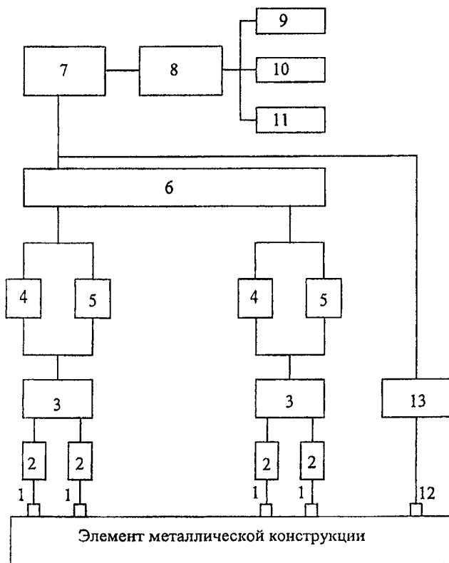
Рис. 6.2.1. Структурная схема АЭ диагностического комплекса:
