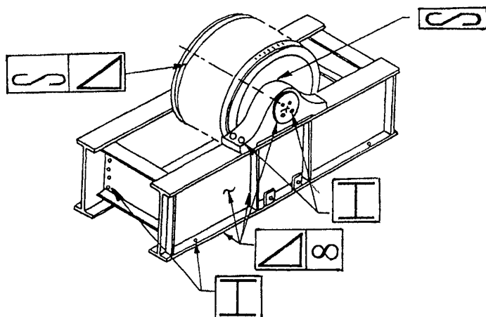
Рис. 5.3. Кронблок
