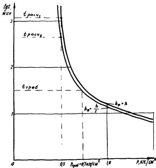
Рис.2. Зависимость времени достижения \lambda_{расч} = 0.3 от нагрузки
