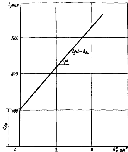
Рис.3. Зависимость времени достижения расчетной относительной деформации от квадрата высоты образца
