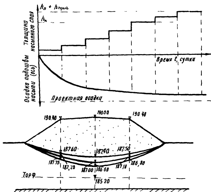
Рис.4. Регистрация положения подошвы насыпи по результатам нивелировки
