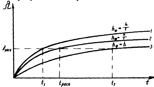
Рис.3. Расчетные кривые консолидации для определения консолидационных характеристик: 1-двустороннее отжатие воды; 2-то же; 3-одностороннее отжатие воды
