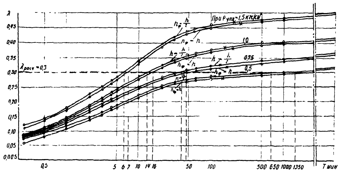
Рис.1. Кривые консолидации \lambda = f(t_{qT}) (торф с участка автомобильной дороги Москва-Изма при h = 2 \text{ см}
