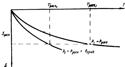
Рис.1. Зависимость времени T достижения заданной осадки S' от величины действующей нагрузки P
