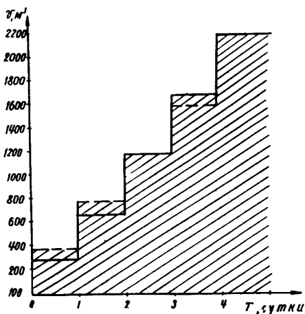
Рис.5. График фактического режима отсыпки насыпи
