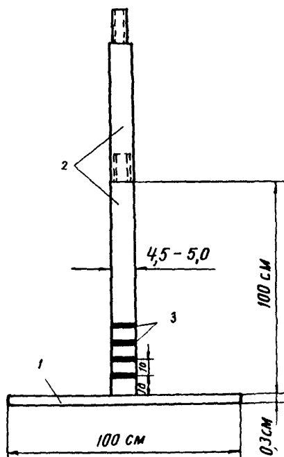
Конструкция осадочной марки
