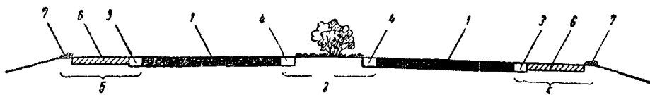
Рис. 2. Основные элементы поперечного профиля автомагистрали: 1— проезжая часть; 2— разделительная полоса; 3— внешняя краевая полоса; 4— внутренняя краевая полоса; 5— обочина; 6— укрепленная часть обочины (стояночная полоса или дополнительная полоса для движения на подъем); 7— грунтовая обочина.
