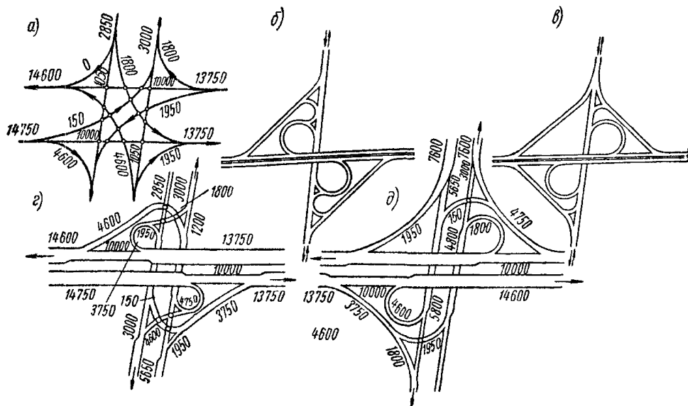
Рис 12 Варианты пересечения по типу неполного клеверного листа:
