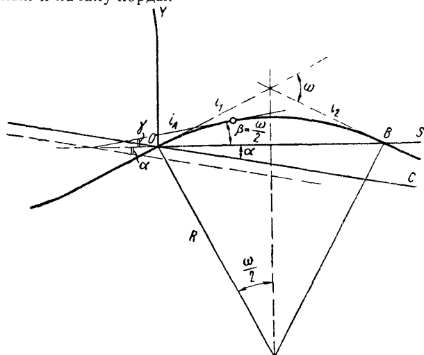
Рис. 4. Схема к выводу уравнения движения автомобиля по вертикальной кривой.
