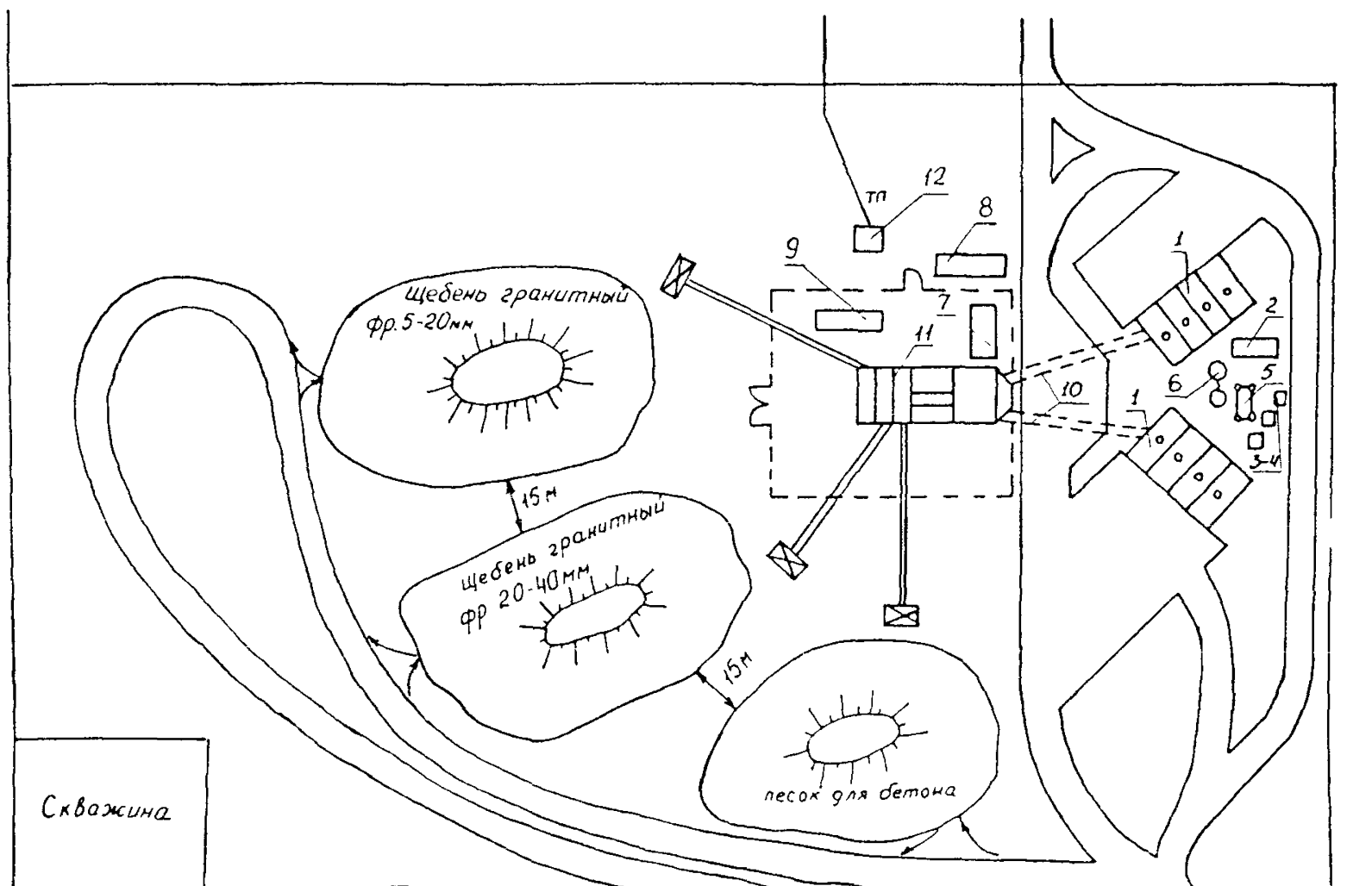
Рис. 1. План размещения завода «Рекс»:
