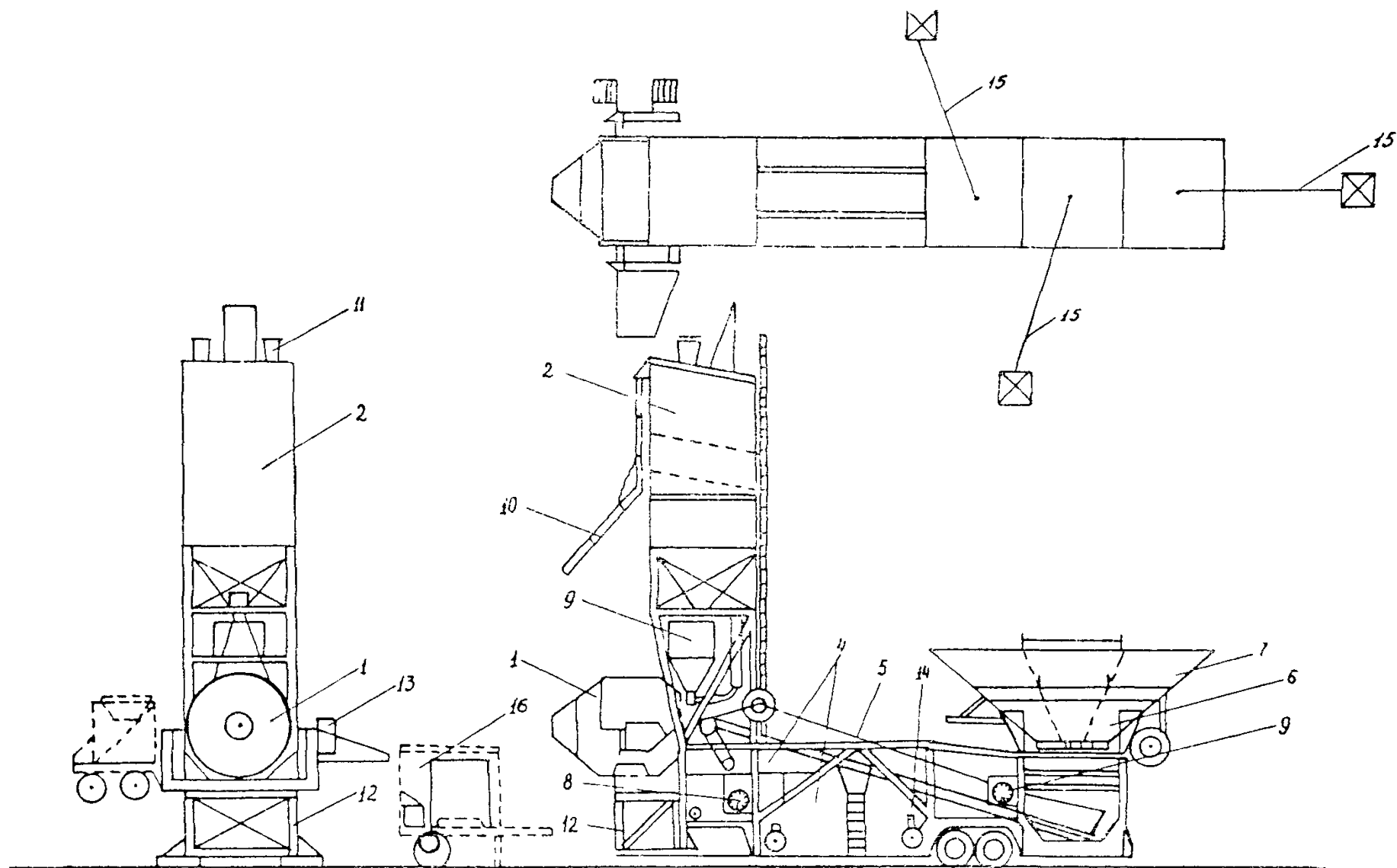
Рис. 2. Схема установки «Рекс».
