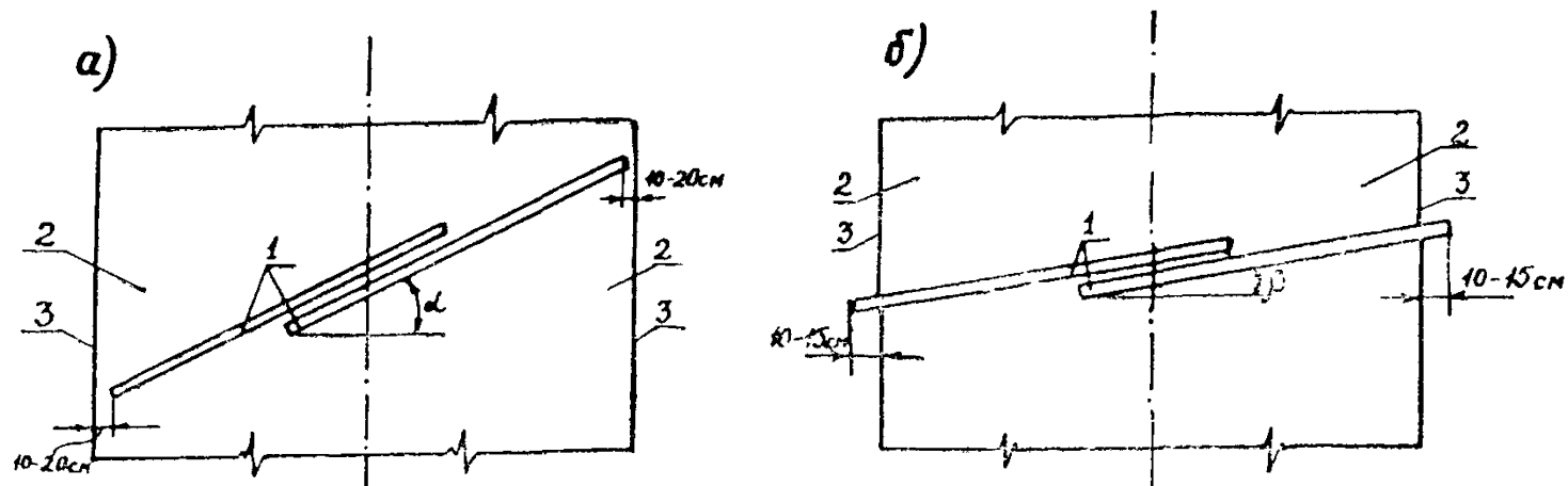
Рис. 1. Положение выравнивающих труб при работе трубного финишера ТФВ-280 а—при предварительной отделке поверхности бетона, б—при окончательной отделке поверхности бетона; 1—выравнивающие трубы, 2—цементобетонное покрытие; 3—кромка покрытия, \alpha —угол поворота труб при предварительной отделке; \beta —угол поворота труб при окончательной отделке поверхности покрытия
