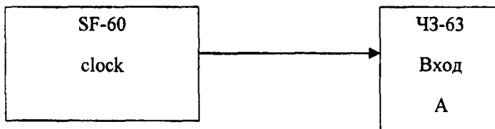
Рисунок 1. Проверка тактовой частоты
