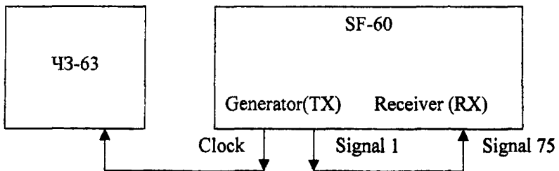
Рисунок 3. Проверка погрешности индикации сдвига частоты
