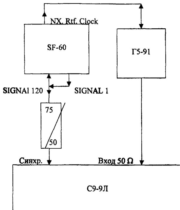
Рисунок 7. Проверка погрешности установки амплитуды джиттера на скоростях 2048, 34368 и 139264 кбит/с
