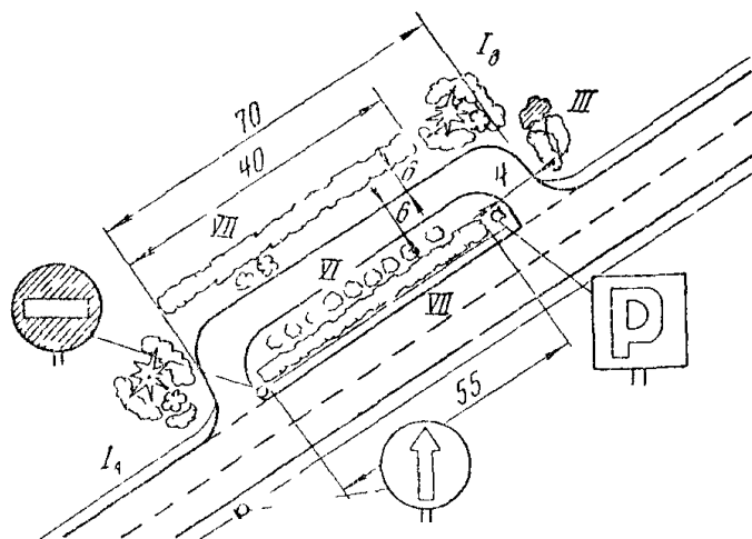
Рис. 26,а Пример планировки площадок отдыха в пределах обреза полосы отвода
