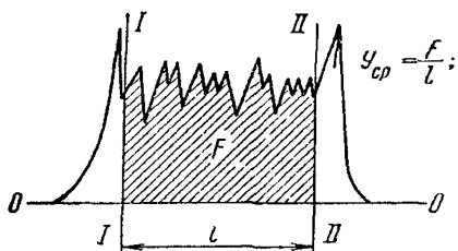
Рис. 67. Образцы записи коэффициента сцепления
