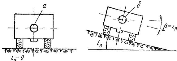
Рис. 24. Схема определения поперечного уклона с помощью гироскопических датчиков
