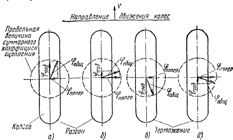
Рис. 22. Соотношение используемых коэффициентов сцепления в продольном и поперечном направлениях при \varphi_{\text{общ}} = \text{const} , но при различных условиях движения
