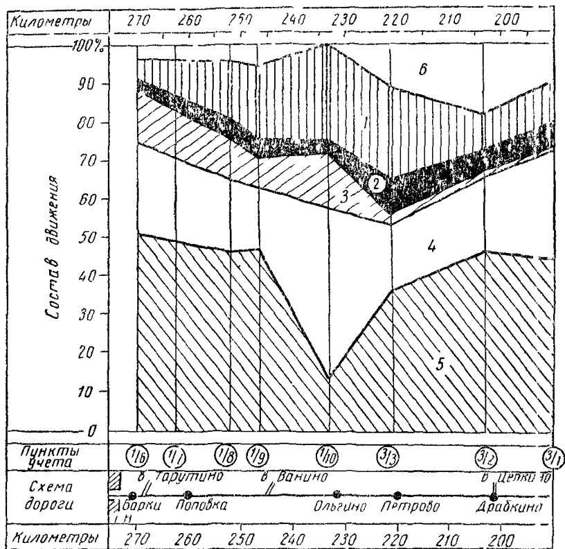
Рис 8 Линейный график изменения состава движения по дороге 1 — легковые автомашины, 2 — автобусы, 3 — грузовые тяжелые автомобили, 4 — грузовые средней грузоподъемности, 5 — грузовые малой тоннажа, 6 — прочие автомобили
