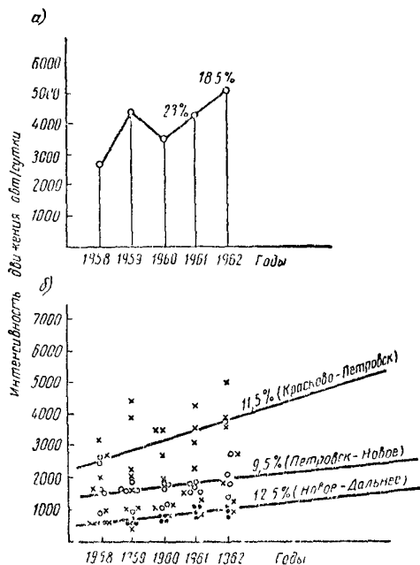
Рис. 12. Определение темпов роста интенсивности движения
