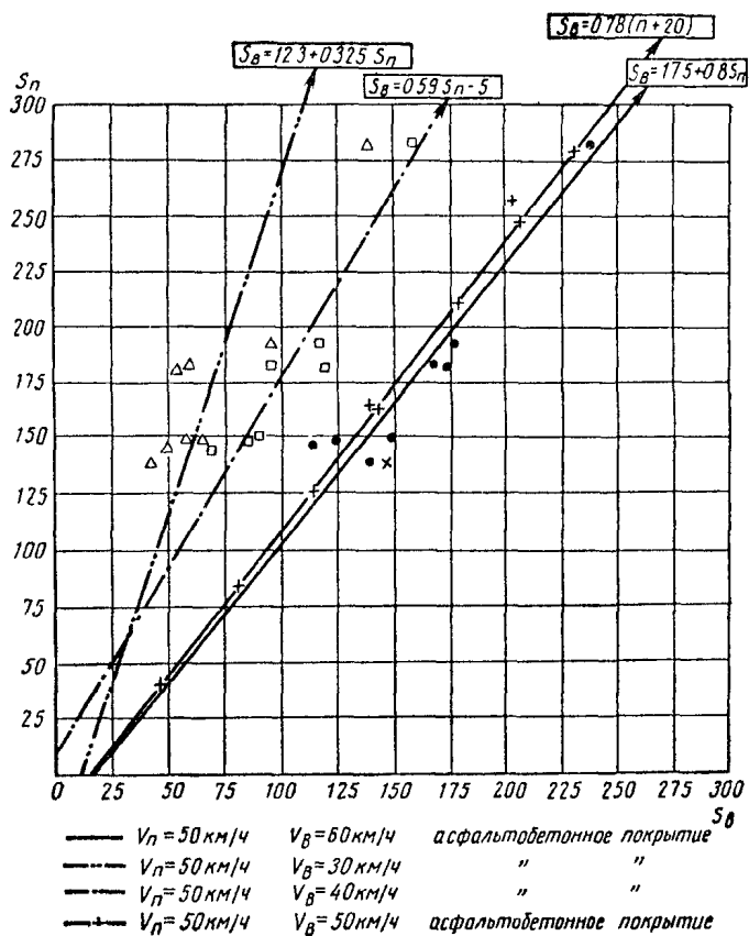
Рис 62. График зависимости показаний толчкометров, установленных на автомобилях М-21 «Волга» (МАДИ) и М-20 «Победа» (ХАДИ)
