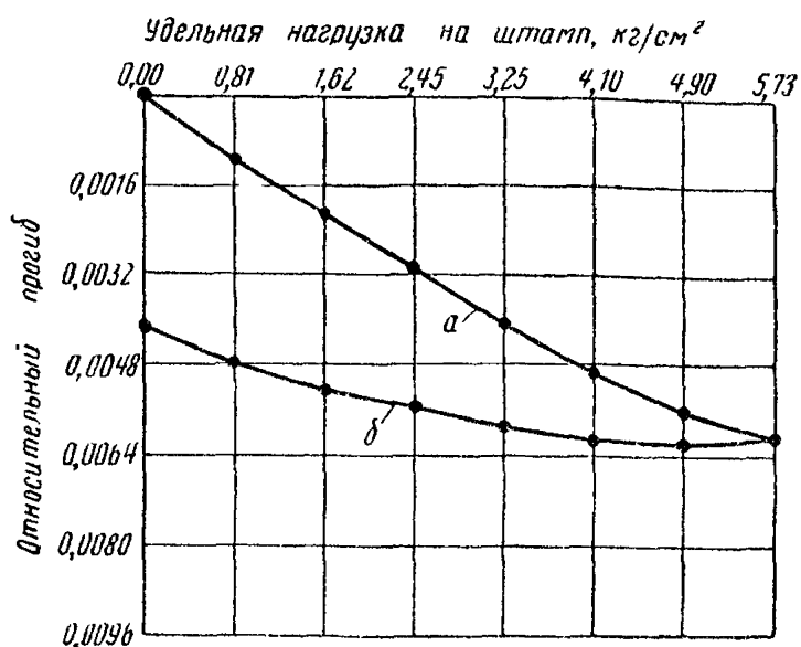
Рис. 56. Результаты оценки прочности дорожной одежды вдавливанием штампа a — везьв нагружения, б — везьв разгрузки
