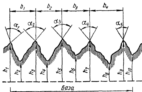
Рис 64 Основные характеристики шероховатости h — высота неровности b — шаг (неровности (расстояние между выступами) \alpha — угол при вершине
