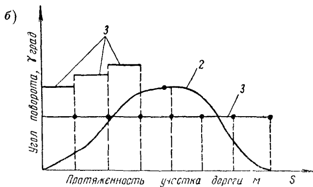
Рис 20,а Обработка записей режимов движения на осциллограф Построение графика кривизны в функции пути
