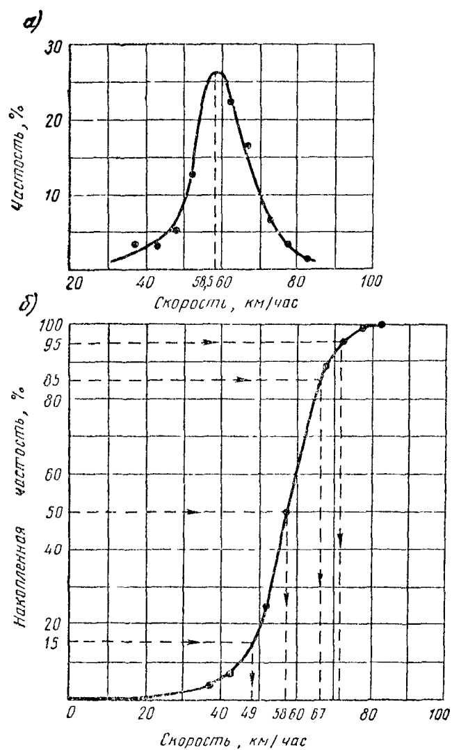
Рис 34 Статистическая обработка результатов наблюдения
