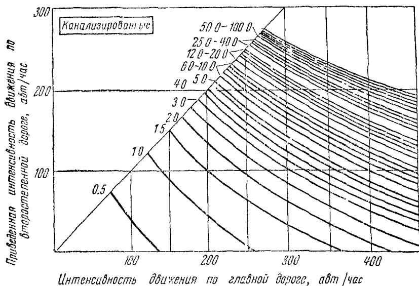
Рис. 42. Потери времени на канализированных транспортных узлах в одном уровне в зависимости от интенсивности движения на пересекающихся дорогах
