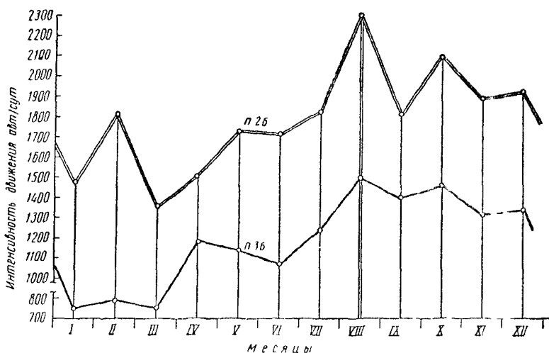
Рис. 11 Годовой график изменения интенсивности движения на двух учетных пунктах
