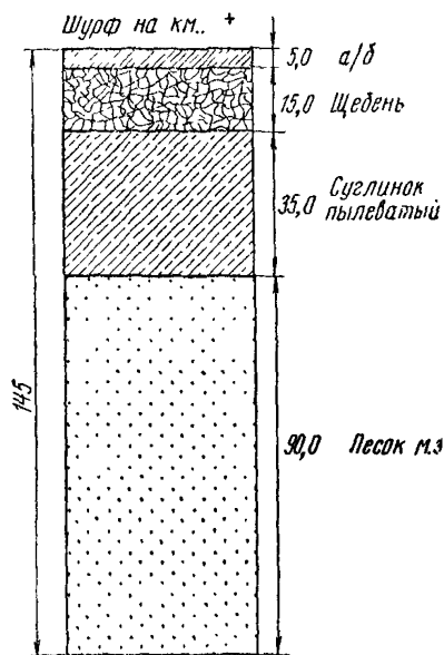
Рис. 47. Разрез шурфа
