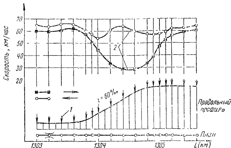
Рис. 32. Расположение створов при измерении мгновенных скоростей на участке подъема 1 — створы, 2 — эпюры скоростей движения
