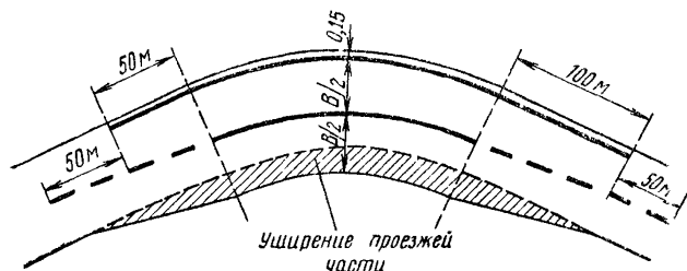
Рис 45 Общий вид разметки, ограничивающей скорость входа автомобилей на кривую
