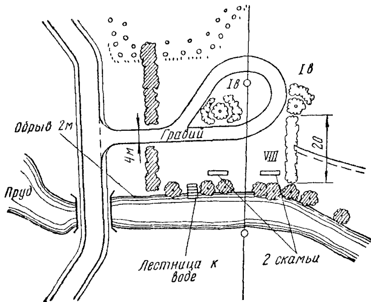
Рис. 26,б. Площадка туикового типа, расположенная у живописного места и требующая дополнительного отвода земель
