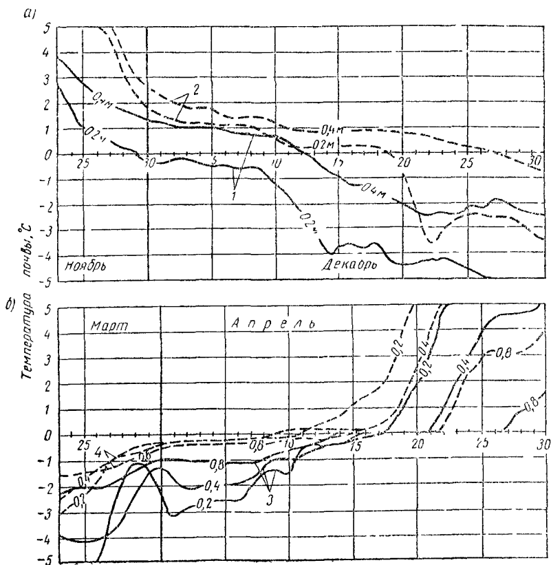
Рис. 5. Ежедневные средние температуры почвы в районе обследуемой дороги на различных глубинах
