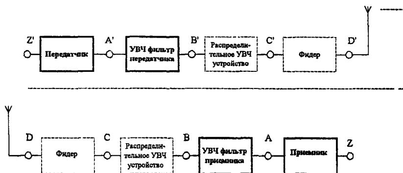
Рисунок 5.2 - Структурная схема радиооборудования APД FH-CDMA 3-11 ГГц
