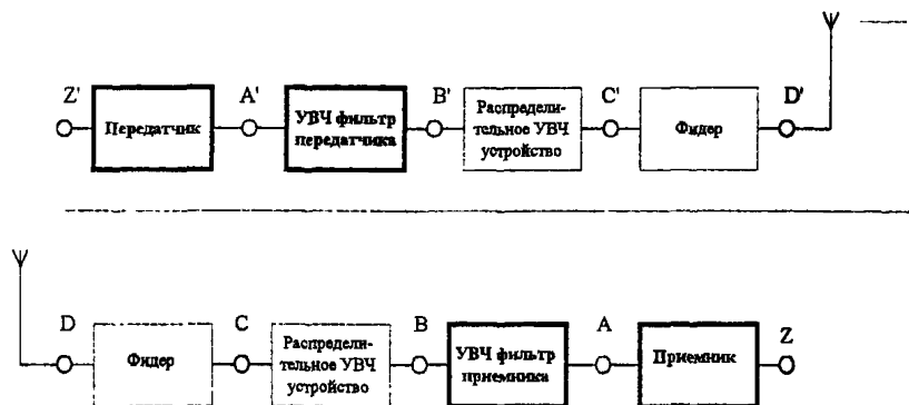
Рисунок 5.2 - Структурная схема радиоборудования APД FH-CDMA 1-3 ГГц
