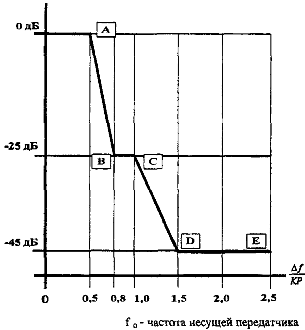
Рисунок 5 3 - Зависимость относительных уровней ограничительной линии спектра от \Delta f = f - f_0 для различных значений канального разнеса (КР)
