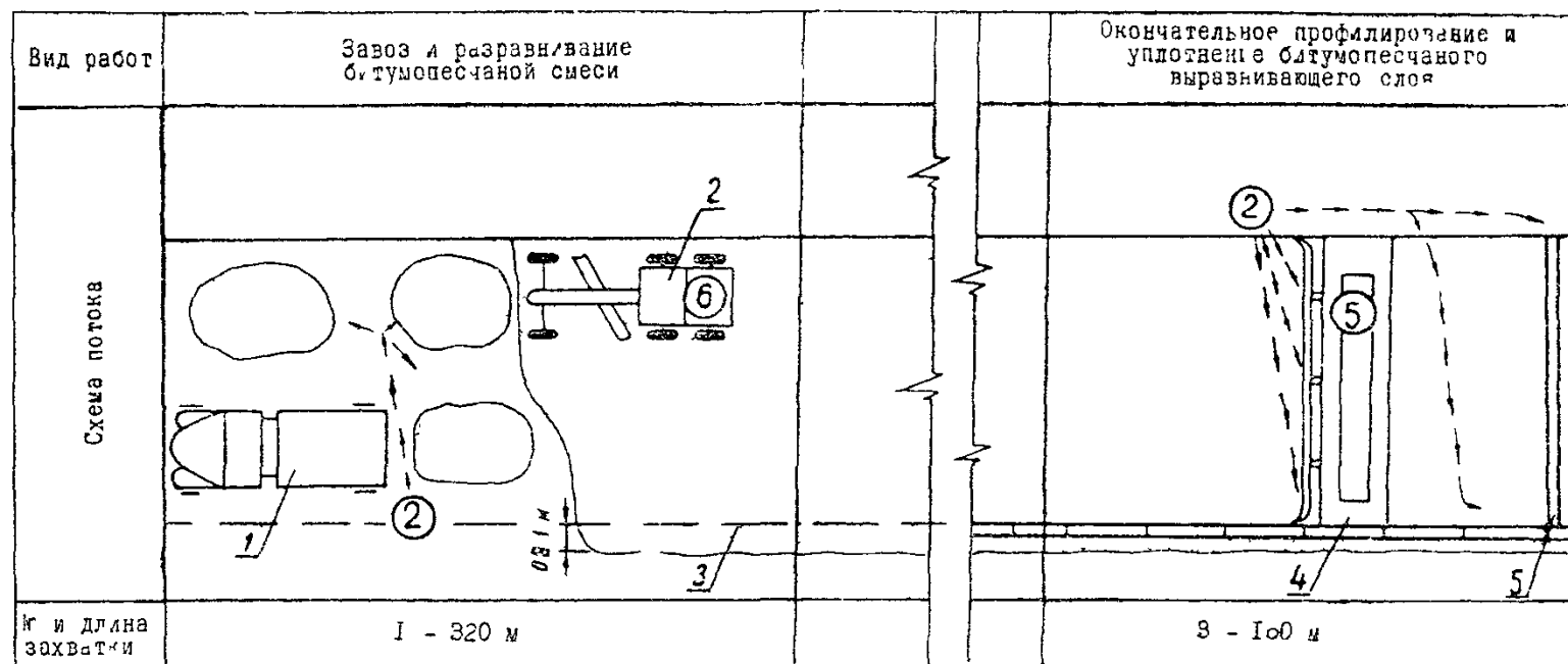
Рис 1 Технологическая схема устройства битумно песчаного выравнивающего слоя 1—автомобиль самосвал 2—автогрейдер Д 144 3—линия установки рельс форм 4—профилировщик Д-345, 5— шаблон для проверки поперечного профиля выравнивающего слоя Кругами с цифрами обозначены рабочие и их разряд стрелками—перемещения рабочих в течение смены
