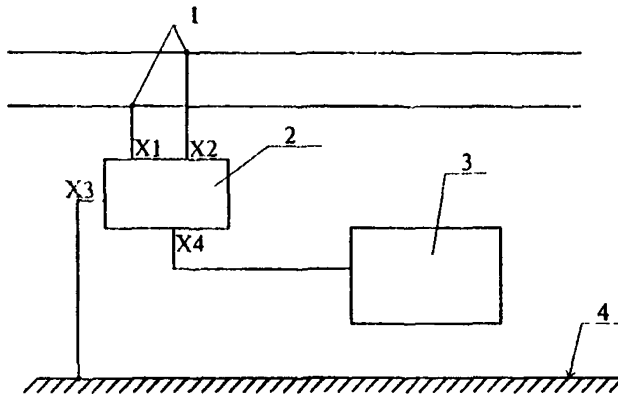
1 - зажимы на двухпроводной симметричной линии связи; 2 - Т-образный эквивалент сети; 3 - измеритель радиопомех; 4 - "земля"
