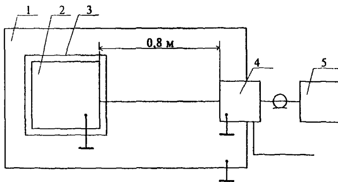
1 - металлический лист; 2 - испытуемое оборудование; 3 - подставка из изоляционного материала; 4 - эквивалент сети; 5 - измеритель радиопомех
