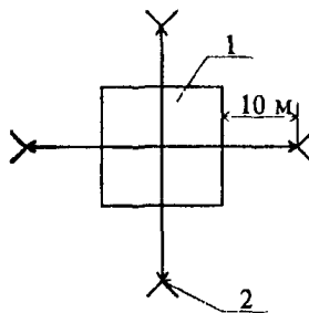
1 - испытуемое оборудование; 2 - положение антенны при испытаниях.
