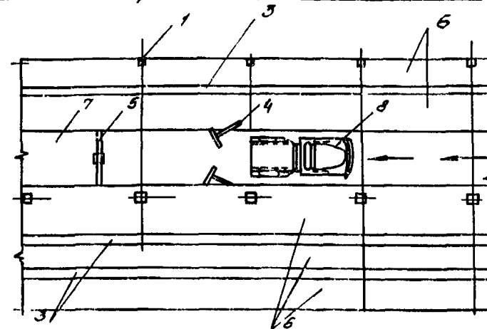
Схема бетонирования с помощью самосвала
