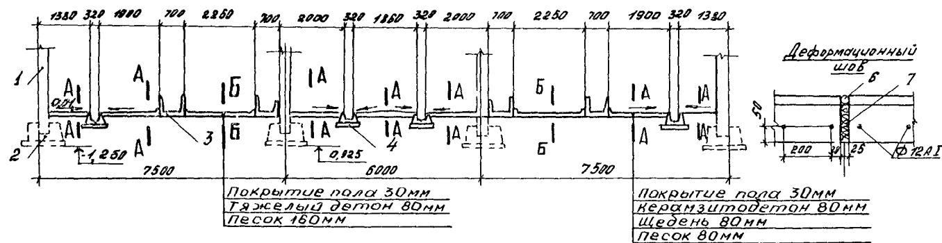
Разрез 1-1
