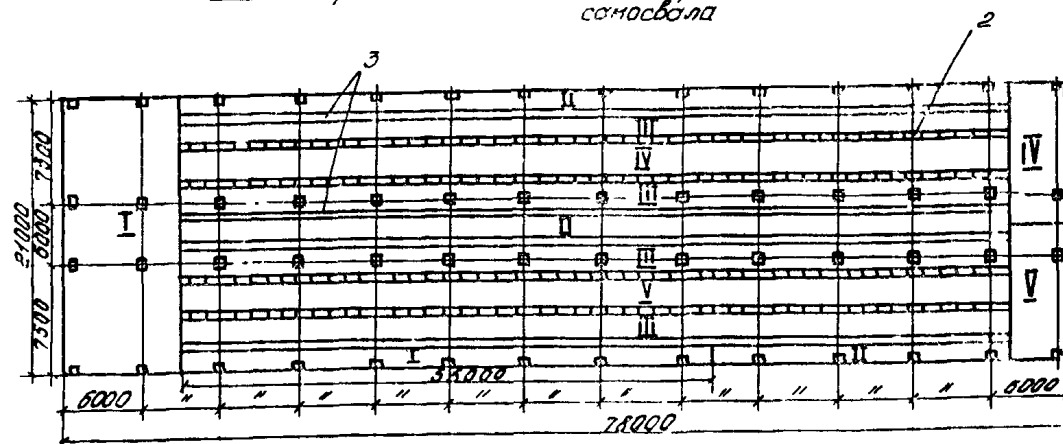
Схема разбивки на захватки при бетонировании с помощью самосвала
