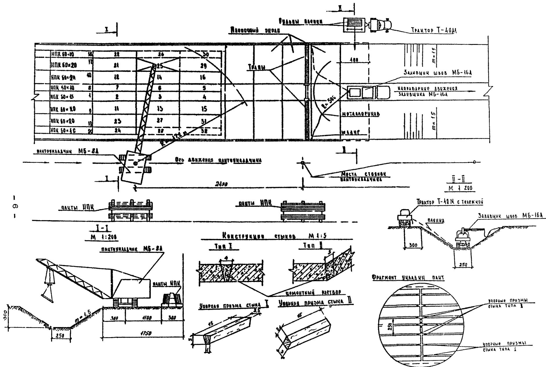
Рис. 3. Схема устройства пленочного экрана и монтажа плит
