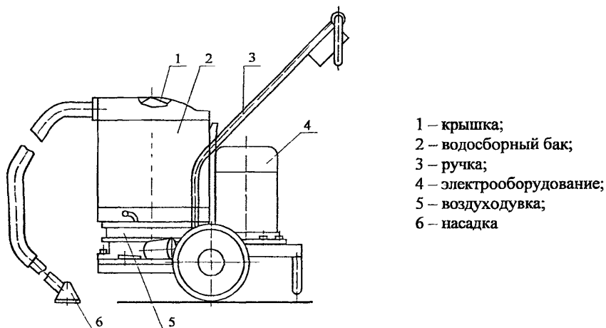
Рисунок 2 – Машина СО-16А для удаления влаги с изолируемой поверхности
