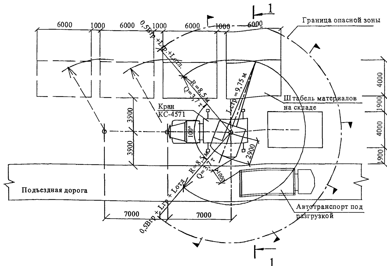
Рисунок 16 – Горизонтальная привязка крана KC-4571
