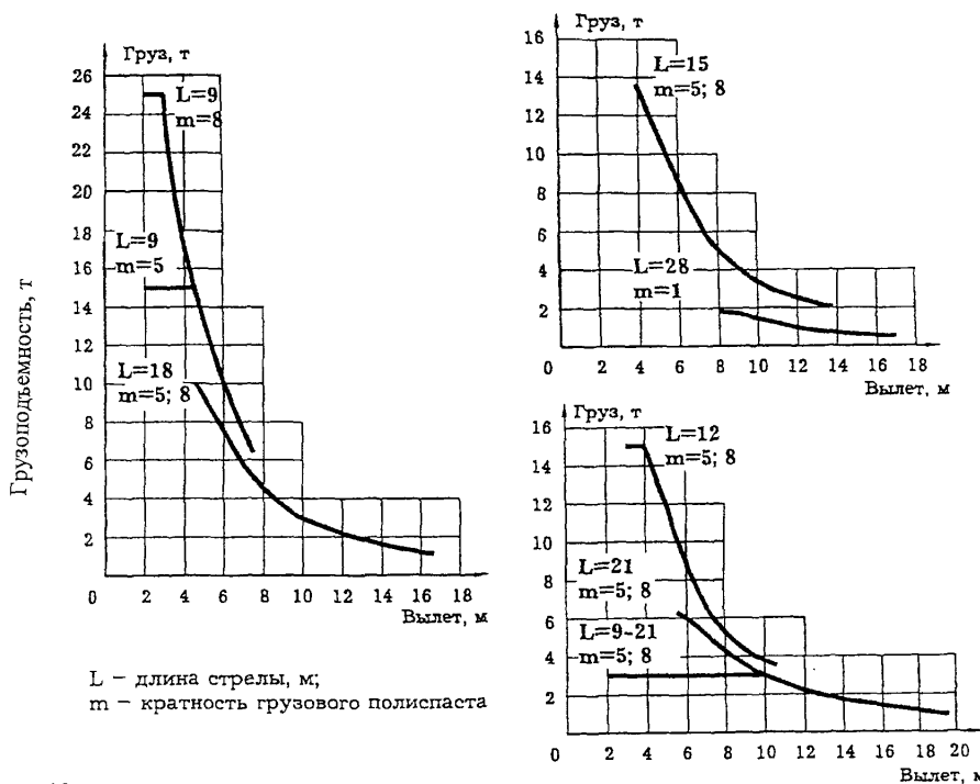
Рисунок 19 – Грузовые характеристики крана КС-45717К-1 при работе с обычными грузами (на выносных опорах)
