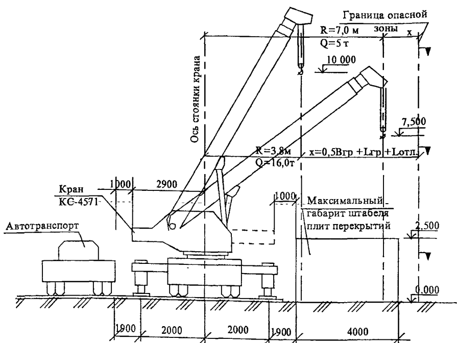
Рисунок 17 – Вертикальная привязка крана KC-4571
