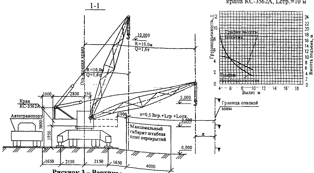
Рисунок 3 – Вертикальная привязка крана КС-3562А (КС-3562Б)
