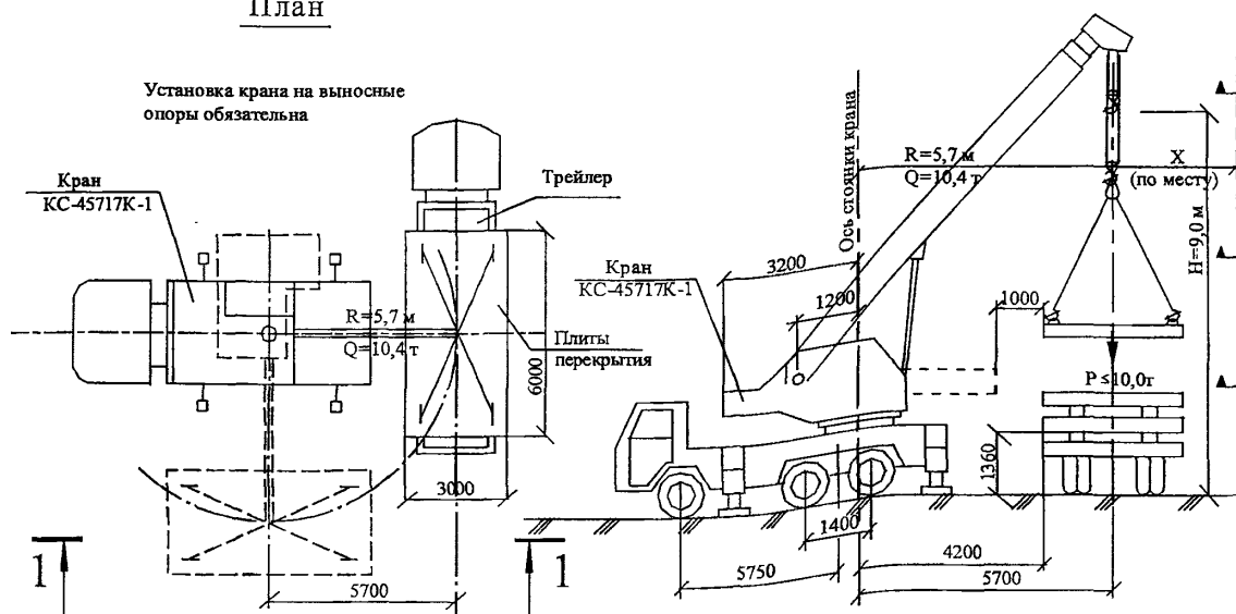
Рисунок 24 – Погрузка и разгрузка плит перекрытия краном KC-45717K-1
