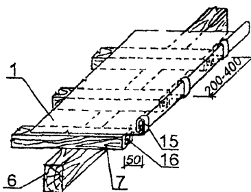
Крепление фронтового края рядовой полосы
