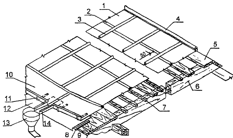
Крепление фронтового края рядовой полосы
