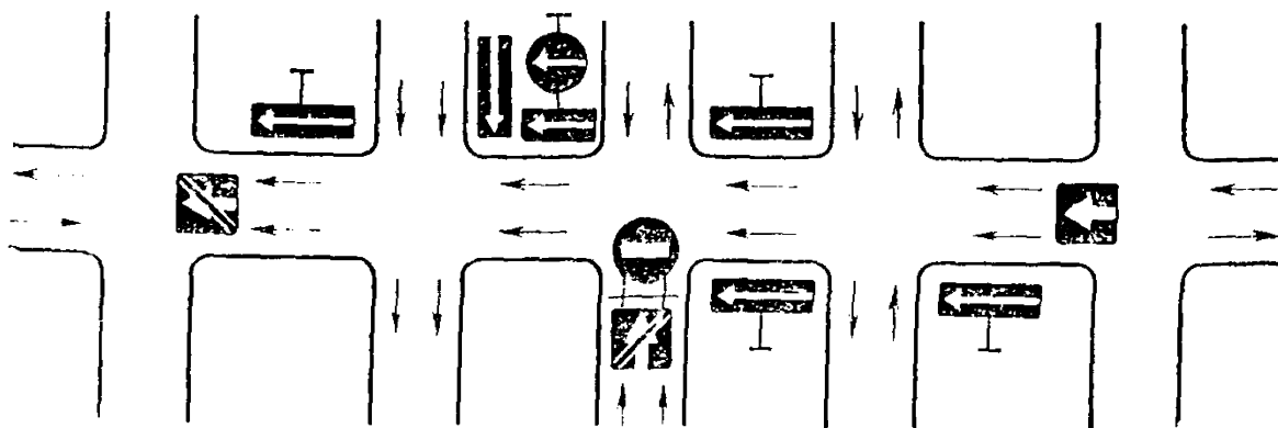
Рис. 8.3. Пример организации одностороннего движения
