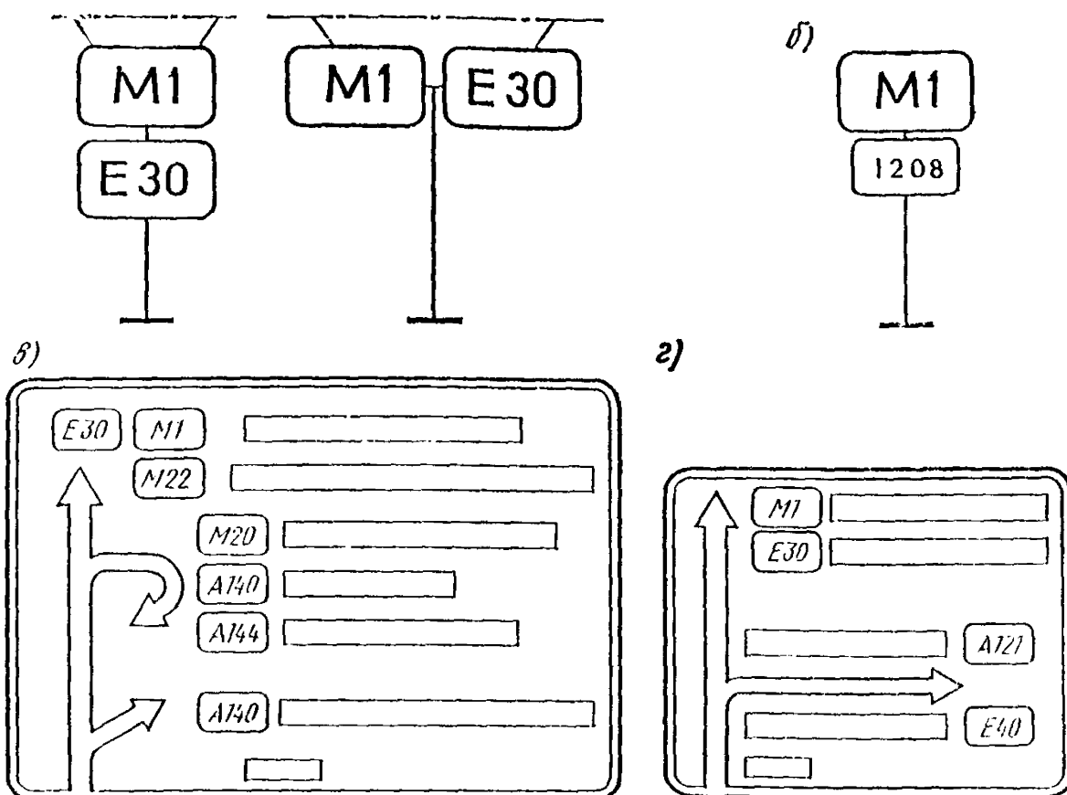
Рис. 19.10. Примеры расположения знаков 5.29.1:
