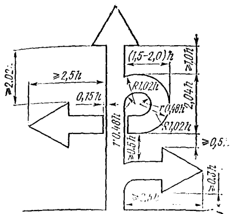
Рис. 19.3. Конфигурация стрелок на знаке 5.20.1, устанавливаемом перед развязкой в разных уровнях (нижняя стрелка может быть расположена под углом 30^\circ к горизонтали). Применение возможно в случае, если количество элементов в надписях менее семи
