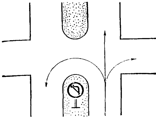
Рис. 7.2. Применение знака 3.18.2 в ситуации, когда не требуется запрещать разворот
