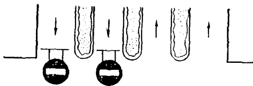
Рис. 6.2. Установка знаков 3.1 при наличии нескольких проезжих частей с односторонним движением
