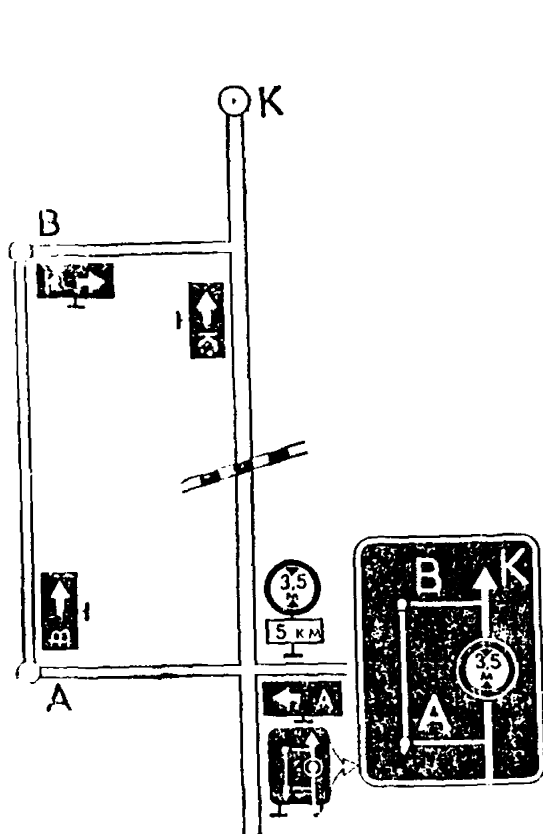
Рис. 12.5. Организация объездного маршрута для транспортных средств, высота которых превышает 3,5 м
