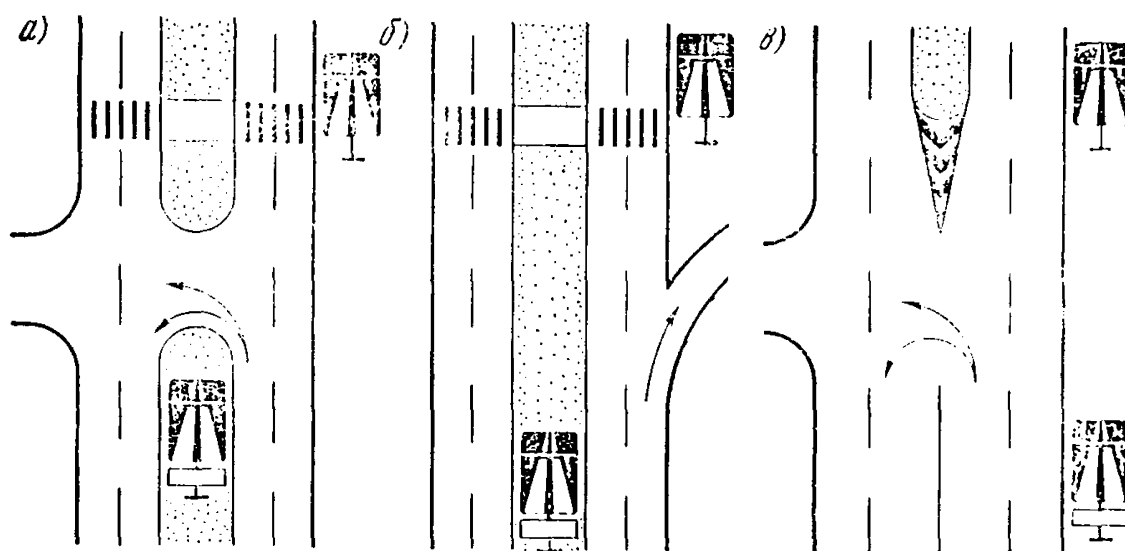
Рис. 8.1. Схемы установки знака 5.1 «Автомобильная»
