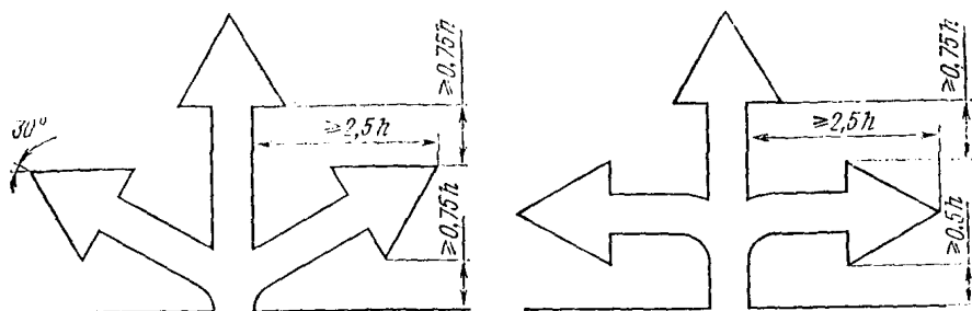
Рис. 19.4. Конфигурация стрелок на знаке 5.20.1, устанавливаемом перед пересечением в одном уровне (возможно сочетание на одном знаке горизонтальной и наклонной стрелок)
