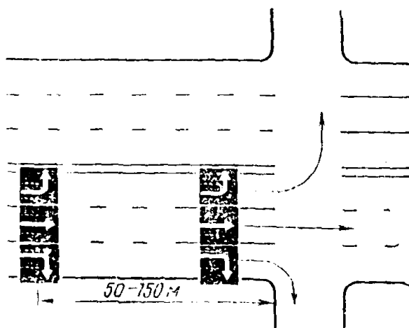
Рис. 8.5. Расположение знаков 5.8.2 относительно перекрестка
