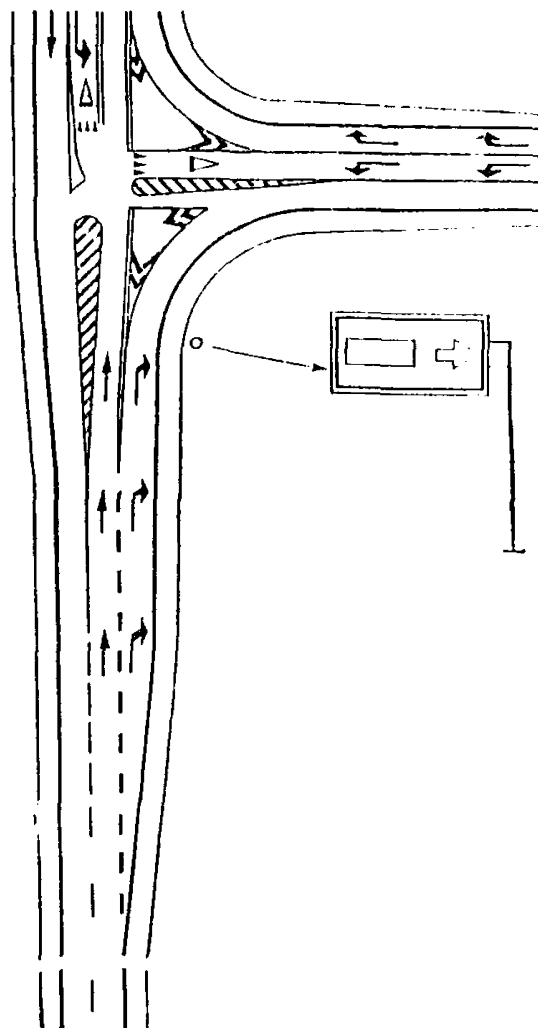
Рис. 13.4. Размещение знака 5.21.2 на Т-образной опоре
