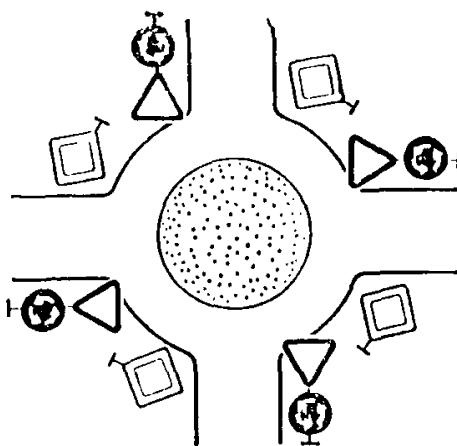
Рис. 13.11. Установка знаков на кольцевом пересечении при предоставлении преимущества транспортным средствам, движущимся по кольцу
