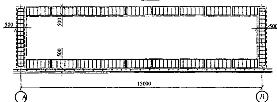
Раскладка армоблоков перекрытия и последовательность монтажа
