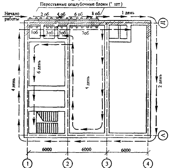
Схема установки опалубки перекрытия
