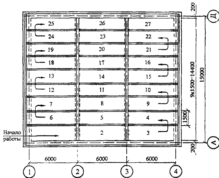
Раскладка арматурных блоков фундаментной плиты и последовательность монтажа
