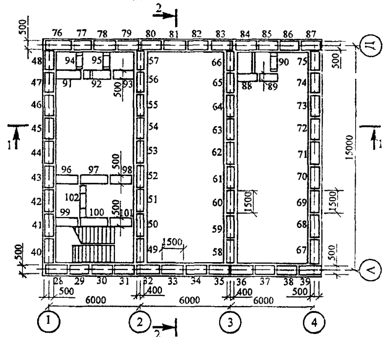
Раскладка арматурных блоков стен и последовательность монтажа
