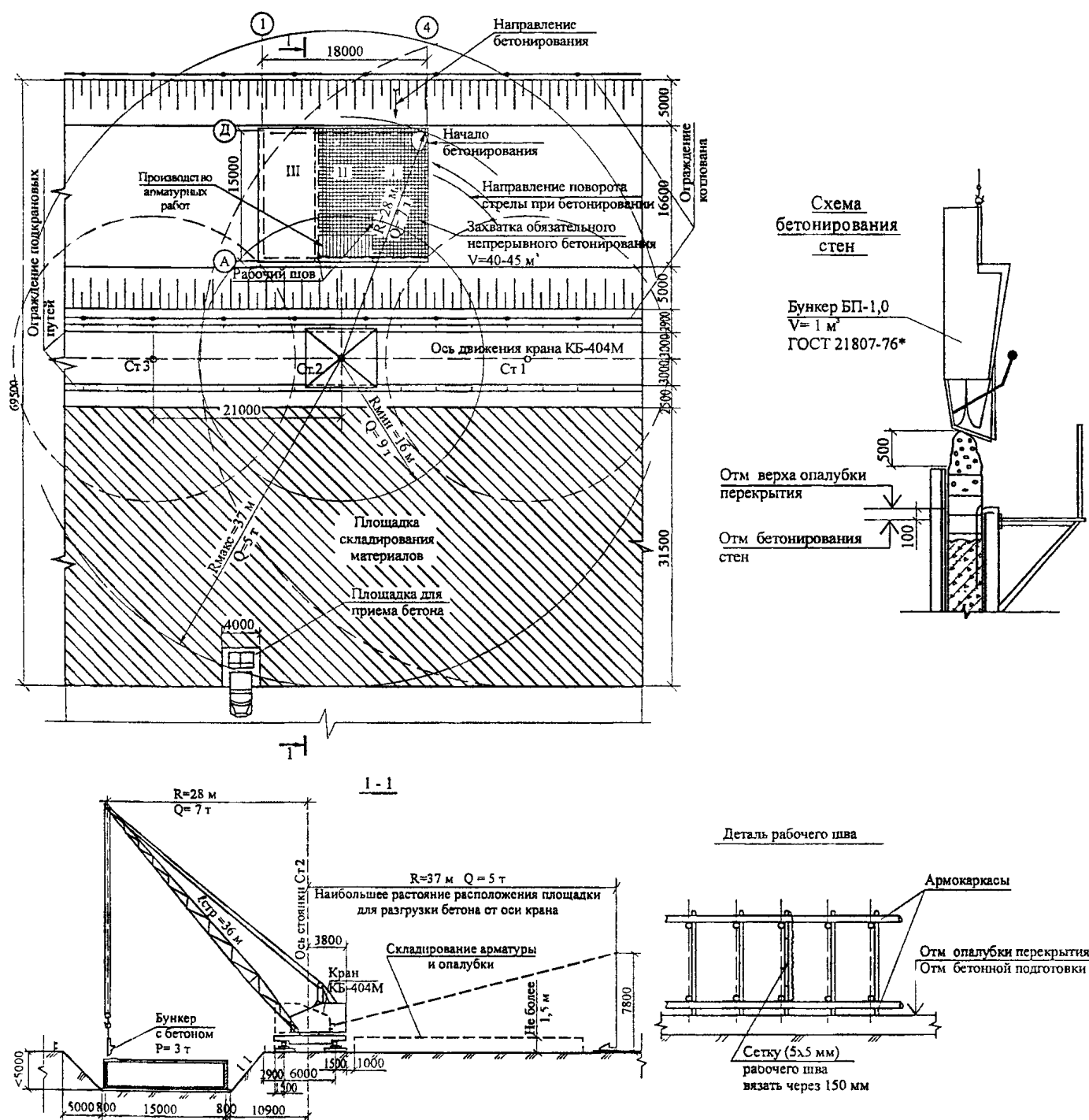
Рисунок 2 – Производство работ при возведении конструкций ГО из монолитного железобетона с помощью крана КБ-404м
