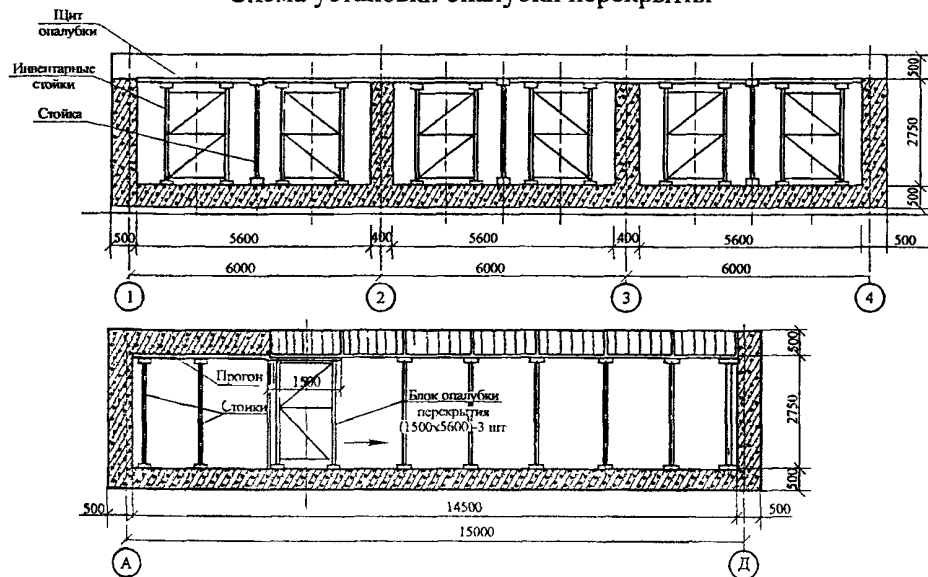
Последовательность укладки бетонной смеси в перекрытие
