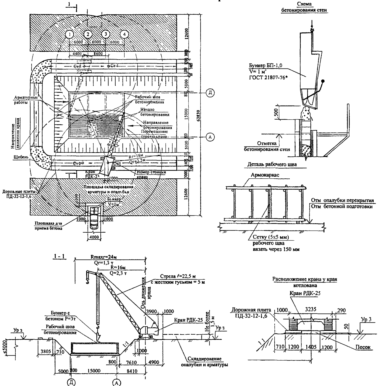
Рисунок 4 – Производство работ при возведении конструкций ГО из монолитного железобетона краном РДК-25
