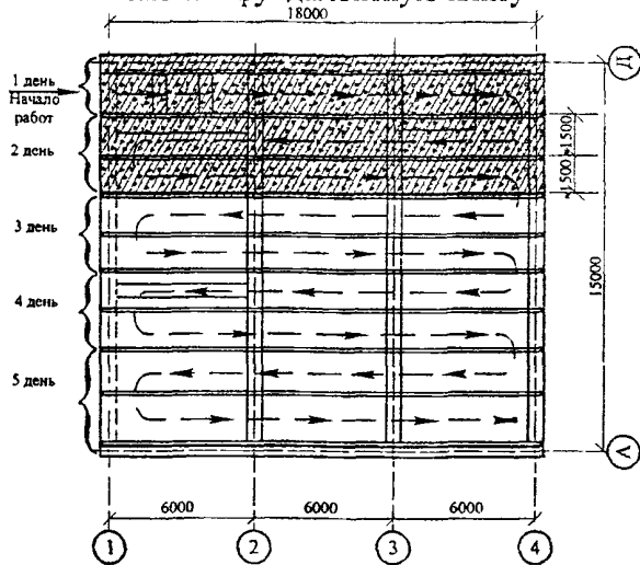
Последовательность укладки бетонной смеси в фундаментную плиту
