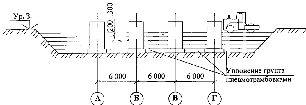
Рисунок 3- Схема послойного уплотнения грунта самоходными катками
