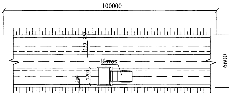
Рисунок-2- Уплотнение грунта при строительстве линейных объектов
