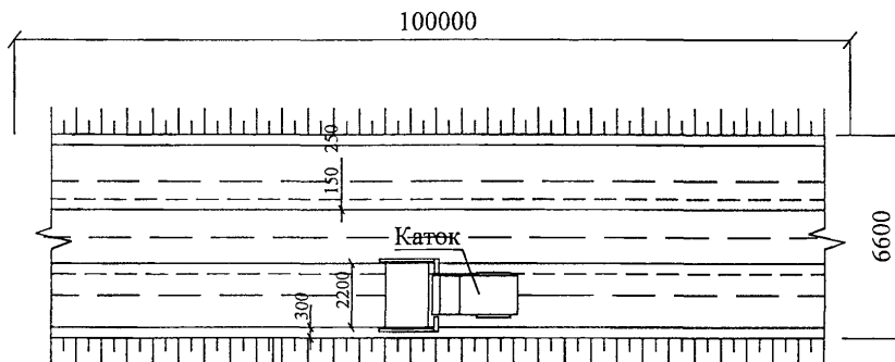
Рисунок 4 – Пример геометрии участка уплотнения для цифровых расчетов
