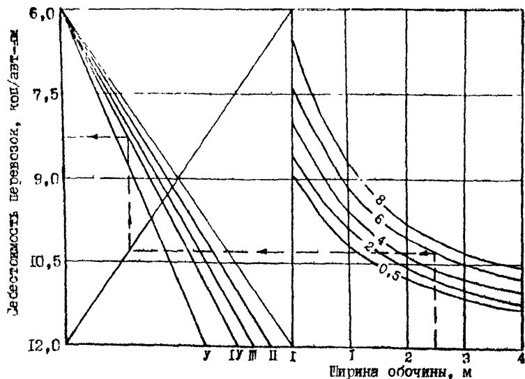
Рис.9.8. Номограмма для определения себестоимости перевозок при различном состоянии обочины /цифры на кривых - интенсивность движения в тыс.авт/сутки/: I - обочины укреплены, имеются краевые полосы, покрытие такое же, как на проезжей части; II - обочины укреплены щебнем, краевые полосы отсутствуют; III - обочины засеяны травой; IV - неукрепленные сухие обочины; V - неукрепленные влажные обочины.
