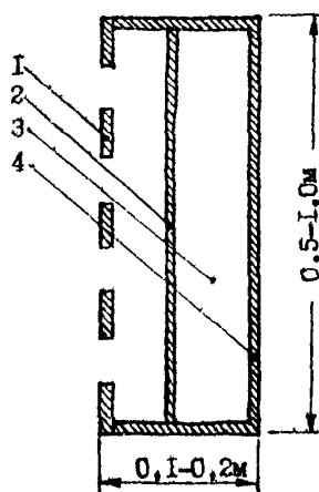
Рис. 5.4. Конструкция элемента шумопоглощающего барьера: 1 - внешняя фронтальная рама; 2 - внутренний поглощающий материал; 3 - слой воздуха; 4 - задняя внешняя рама.
