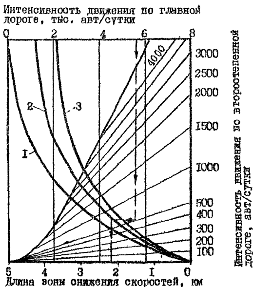
Рис. 9.9. Номограмма для определения протяжения зоны снижения скоростей у пересечений:
