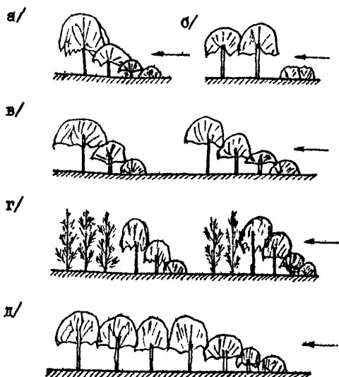
Рис.5.8. Конструкция шумозащитных зеленых насаждений вдоль автомобильных дорог: а - однорядная полоса с плотным прикрыванием крон; б - полоса, не обеспечивающая шумозащиты вследствие распространения звука в подкroновом пространстве; в - двухрядная полоса; г - сочетание лиственных и хвойных пород в шумозащитных полосах; д - однорядная широкая полоса, менее эффективная, чем многорядная той же ширины.
