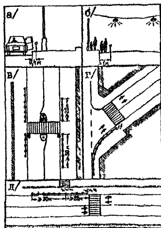
Рис.8.2. Схемы установки ограждений у пешеходных переходов.
