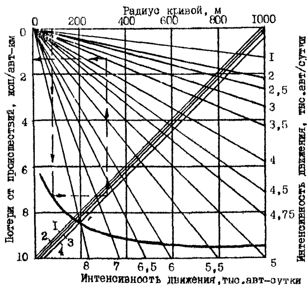
Рис.9.5. Номограмма для определения потерь от дорожно-транспортных происшествий на кривых в плане при различной видимости /расстояние видимости: 1 - более 600 м; 2 - 800 м, 3 - 100 м/.
