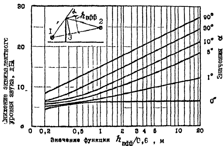
Рис.10.4. Дополнительное снижение эквивалентного уровня звука шумозащитным препятствием: 1 - источник шума; 2 - расчетная точка, 3 - шумозащитное препятствие.
