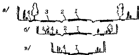
Рис.8.1. Поперечные профили дорог в малых населенных пунктах: а - дорога в насыпи при большой ширине улицы; б - то же при ширине улицы, не позволяющей разместить проезжие части для местного движения; в - поперечный профиль с бордюрами; 1 - проезжая часть дороги; 2 - укрепленные обочины; 3 - проезжая часть для местного движения /при недостаточной ширине улицы может устраиваться с одной стороны дороги/; 4 - тротуары и велосипедная дорожка.
