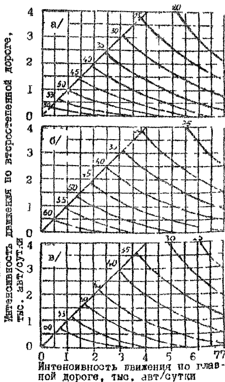
Рис.9.10. Средние скорости движения по главной дороге при различном оборудовании пересечений:
