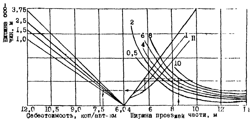
Рис.9.1. Номограмма для определения себестоимости перевозок при различной ширине проезжей части и обочины/цифры на кривых - интенсивность движения в тыс.авт./сутки/: I - краевые полосы по 0,8 м; II - краевые полосы по 0,5
