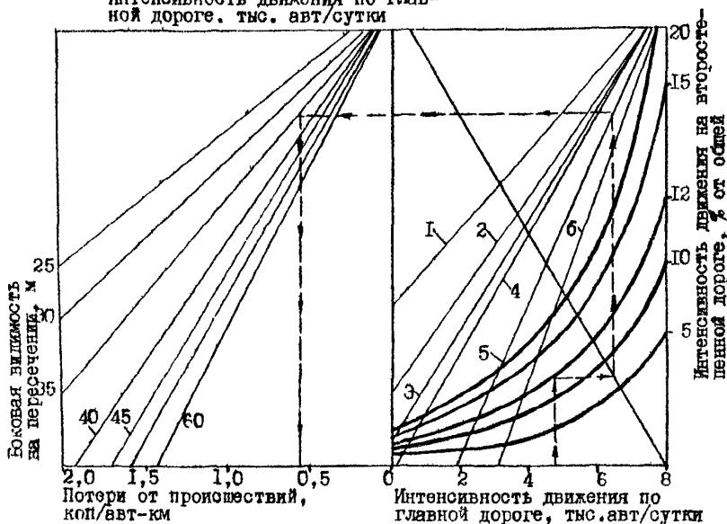
Рис.9.12. Номограмма для определения потерь от дорожно-транспортных происшествий на пересечениях дорог в одном уровне: 1 - пересечение под углом менее 90^\circ ; 2 - примыкание под углом 90^\circ ; 3 - пересечение под углом 90^\circ ; 4 - примыкание под углом 90^\circ ; 5 - пересечение под углом более 90^\circ ; 6 - примыкание под углом более 90^\circ .
