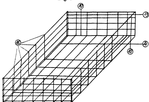
Рис. 3 Наружный каркас прямоугольника № 2
