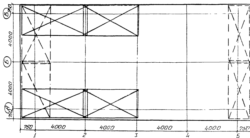
Рис. 6. Схема раскладки сеток С 5
