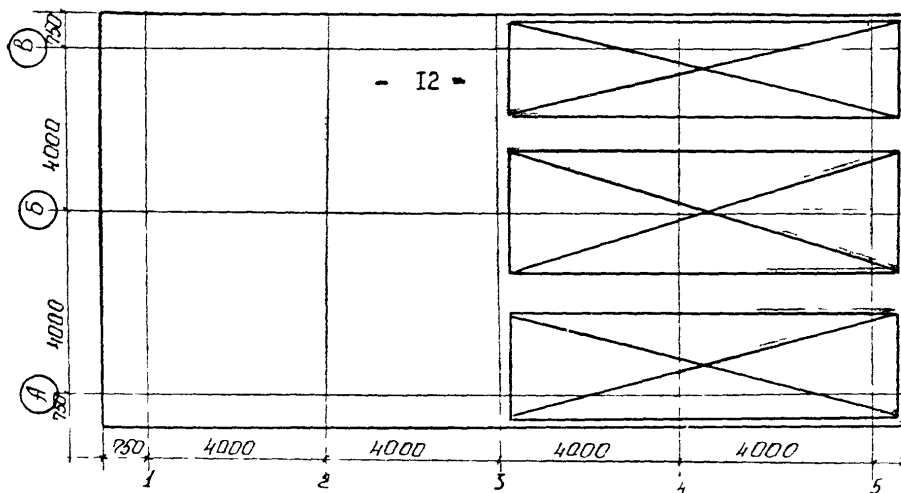
Рис. 8. Схема раскладки сеток C_1 и C_2
