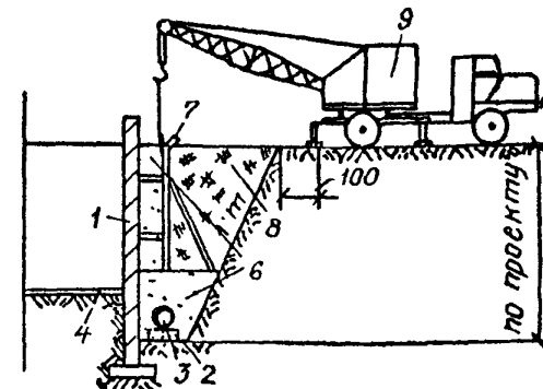
6. Демонтаж щита-опалубки
