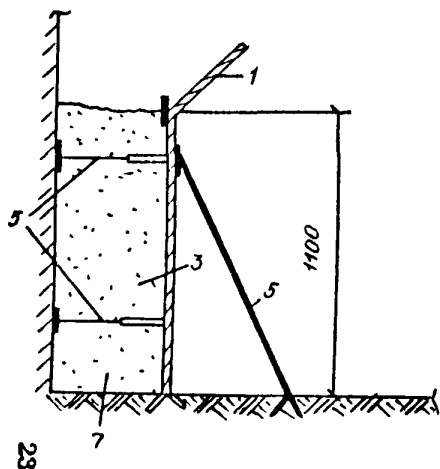
Схема сопряжения щитов-опалубок при их установке
