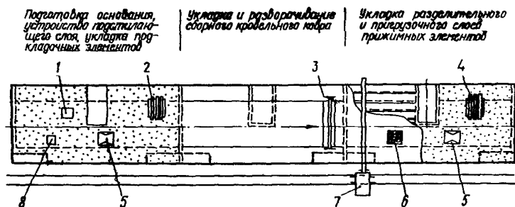
Рис. I. Схема производства кровельных работ: I - контейнер для сыпучих материалов; 2 - поддон с подкладочными сборными железобетонными элементами; 3 - траверса для монтажа сборного ковра; 4 - поддон с прижимными сборными железобетонными элементами; 5 - контейнер для доборных кровельных элементов; 6 - контейнер для рулонных материалов; 7 - башенный кран; 8 - бадья для цементного раствора
