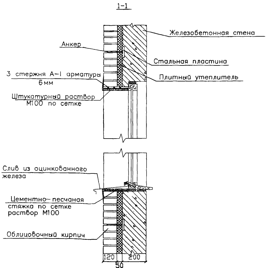
Рисунок 5 – Конструктивное решение облицовки оконных проемов
