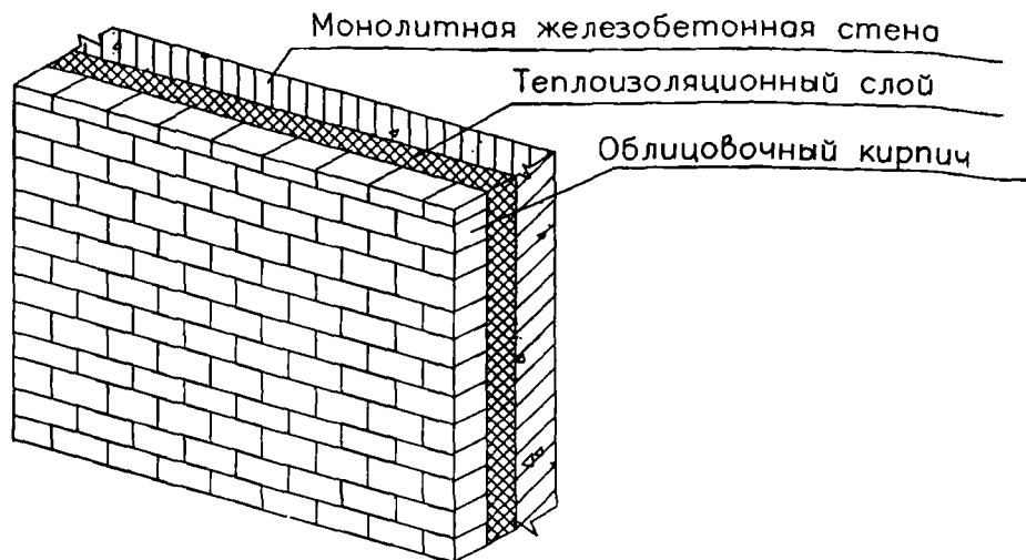
Рисунок 1 – Общий вид стены
