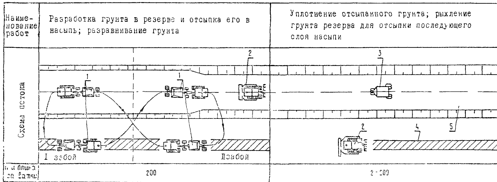
Рис. 1. Технологическая схема возведения земляного полотна:
