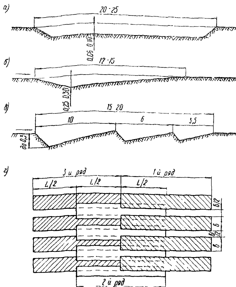
Рис. 2. Схемы зарезания грунта скрепером.
