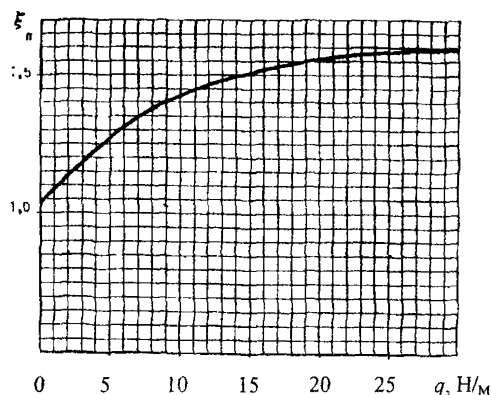
Рис. 2.4. Коэффициент динамичности для проводов контактной сети
