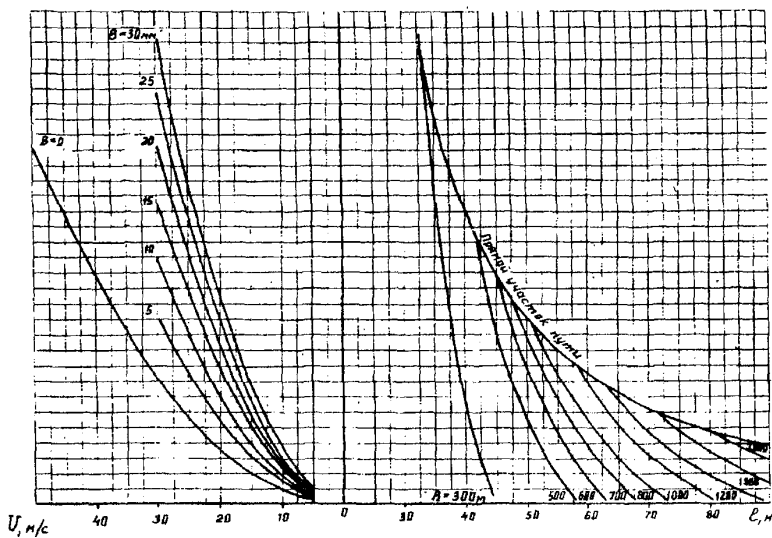
Рис. 2.2. Максимальная допускаемая длина пролетов Переменный ток, подвеска полукомпенсированная, на изолированных консолях: ПБСМ-95+МФ-100, ПБСМ-70+МФ-100
