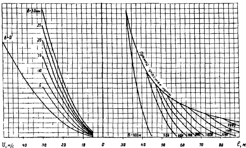
Рис. 2.14. Максимальная допустимая длина пролетов
