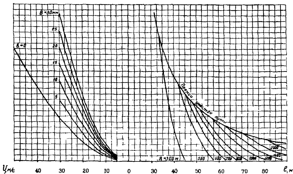
Рис. 2.6. Максимальная допускаемая длина пролетов Переменный ток, подвеска полукомпенсированная на гирлянде из четырех изоляторов ПБСА-50/70+МФ-100
