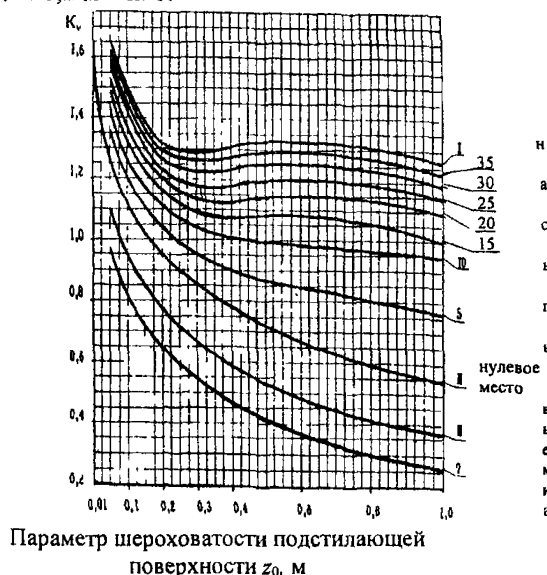
Рис. 2.1. Коэффициент изменения ветрового давления: I — насыпь высотой 40 м ( z_H на рис. 2.2); II — нулевое место; III — выемка глубиной 5 м ( z_B на рис. 2.2)
