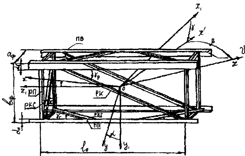
Рис.2.5. Схема отсека фермы
