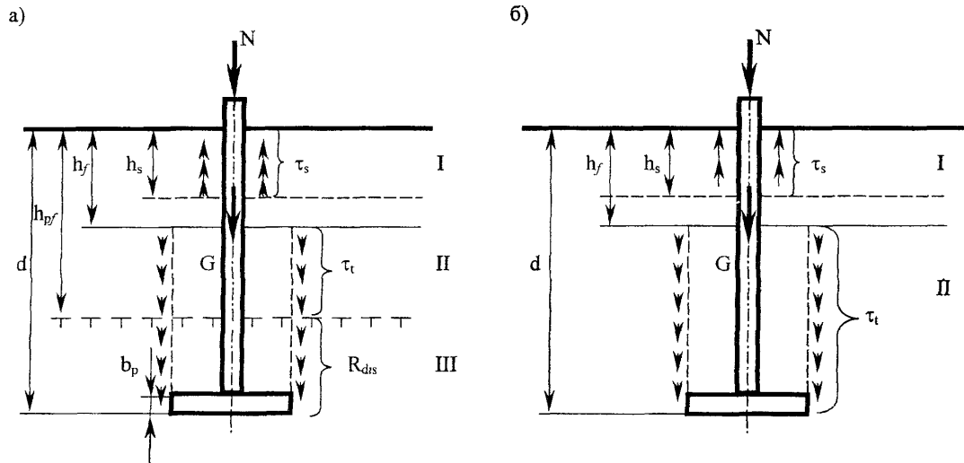
Рис. 7.22. Расчетная схема на выпучивание фундамента с анкерной плитой: а- при заделке фундамента в вечноммерзлый грунт; б- то же в талый грунт; I,II,III- соответственно сезонноммерзлый, талый и мерзлый грунт
