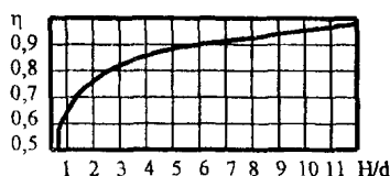
Рис. 7.7 Определение коэффициента \eta , учитывающего влияние плеча N на величину момента
