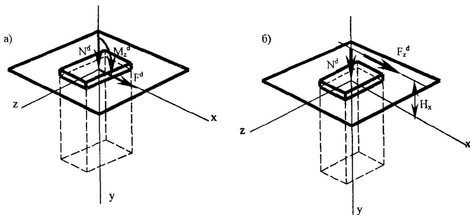
Рис. 7.1. Расчетные схемы нагрузок, действующих в одной плоскости:
