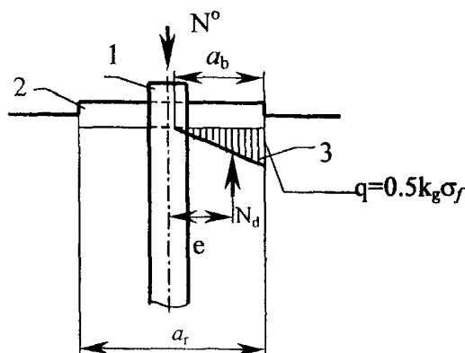
Рис. 7.6 Расчетная схема фундамента с ростверком: 1 - фундамент; 2 - ростверк; 3 - эпюра давления грунта на подошву ростверка
