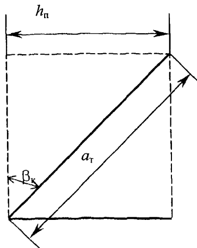
Рис. 2.8 Расположение консоли (в плане) при действии максимальных сил, возникающих при обрыве проводов
