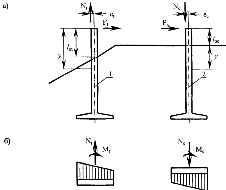
Рис 7 18 Схема сил для расчета прочности раздельного фундамента а – расчетные схемы стоек, б – эпюры реакции грунта, 1 – растянутый блок, 2 – сжатый блок
