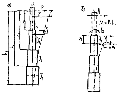
Рис.5.1. Схема опоры с переменным моментом инерции для расчета ее прогибов в точках:
