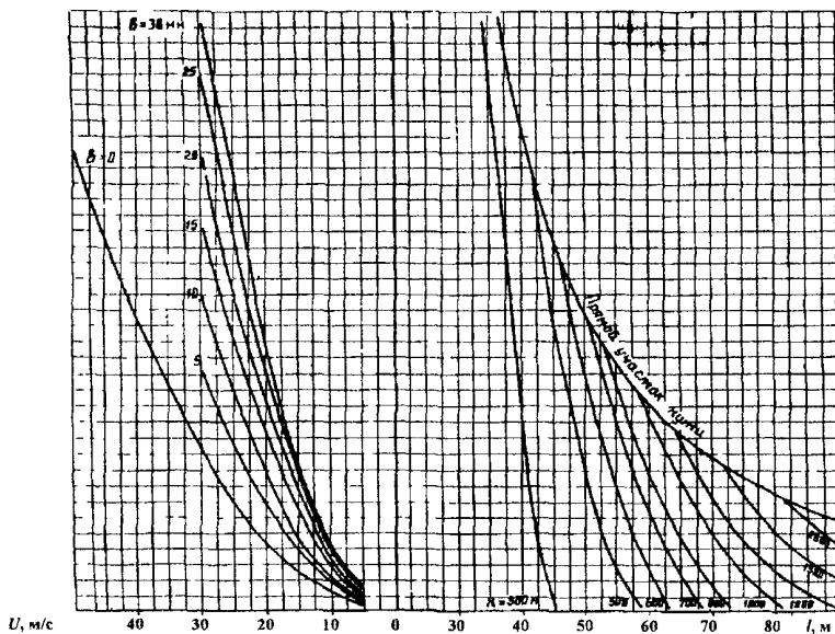
Рис. 2.15. Максимальная допустимая длина пролетов
