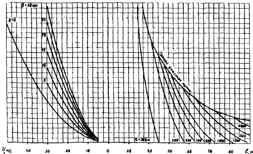
Рис. 2.16. Максимальная допускаемая длина пролетов
