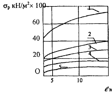
Рис 7.13 Значение \sigma_p для свайного фундамента
