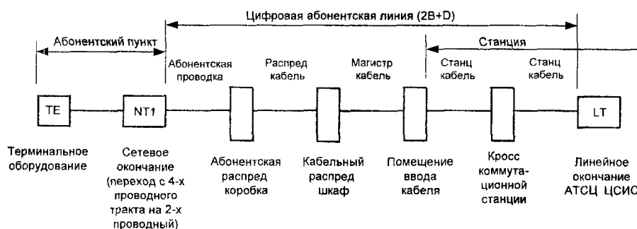
Рисунок 3.1 Структура цифровой абонентской линии (2B+D) ЦСИС
