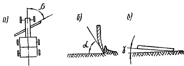
Рис. 3. Углы установки отвала автогрейдера в рабочее положение:
