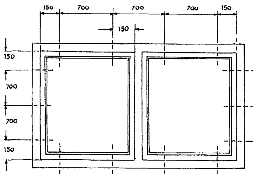
Рис. 3.3. Интервалы крепления
