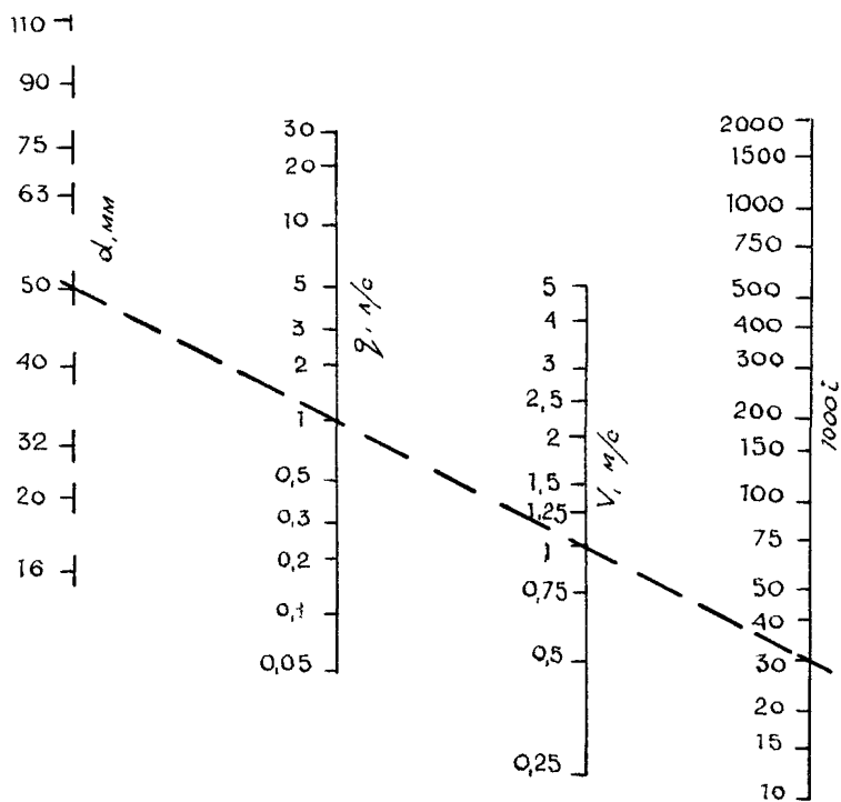
Рис.2. Номограмма для приближенного гидравлического расчета труб ПЭ-х "Профлекс" при средней температуре воды 60°C
