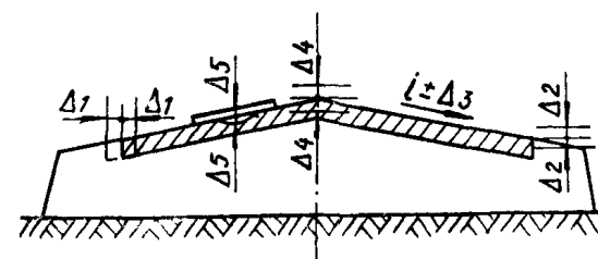
Схема предельных отклонений
