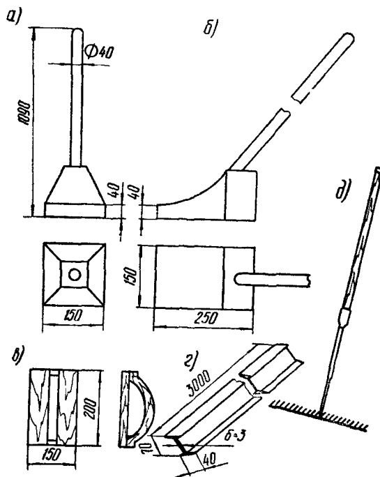
Рис. 2. Инструменты для устройства асфальтобетонных покрытий:
