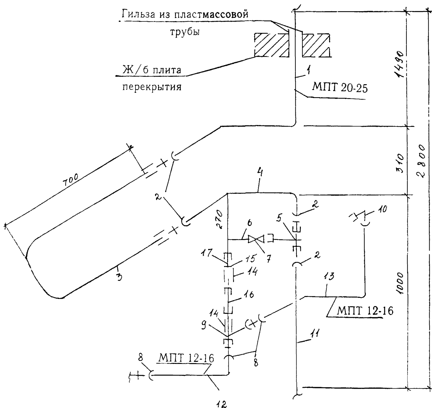
Рис.2. Схема горячего водоснабжения из МПТ:
