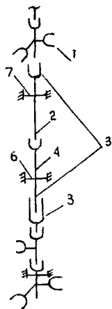
Рис.14. Схема поэтажной сборки канализационного стояка из полипропиленовых труб и фасонных частей:
