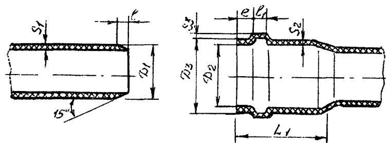
Рис.1. Основные размерные характеристики трубной продукции из ПП
