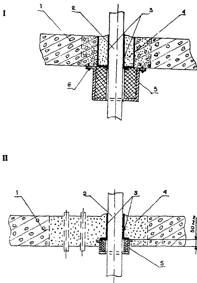
Рис. 36. Схемы конструкции узла прохода канализационного этажа стояка из полипропиленовых труб сквозь железобетонное перекрытие с использованием противопожарной муфты «ОГРАКС-ПМ»:
