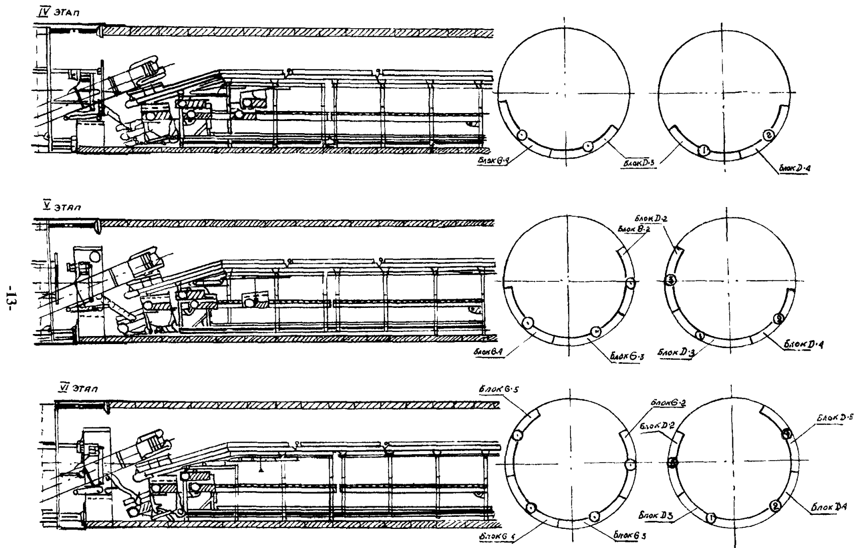
Рис. 7. Последовательность сборки кольца обделки тоннеля. Этапы IV, V, V
