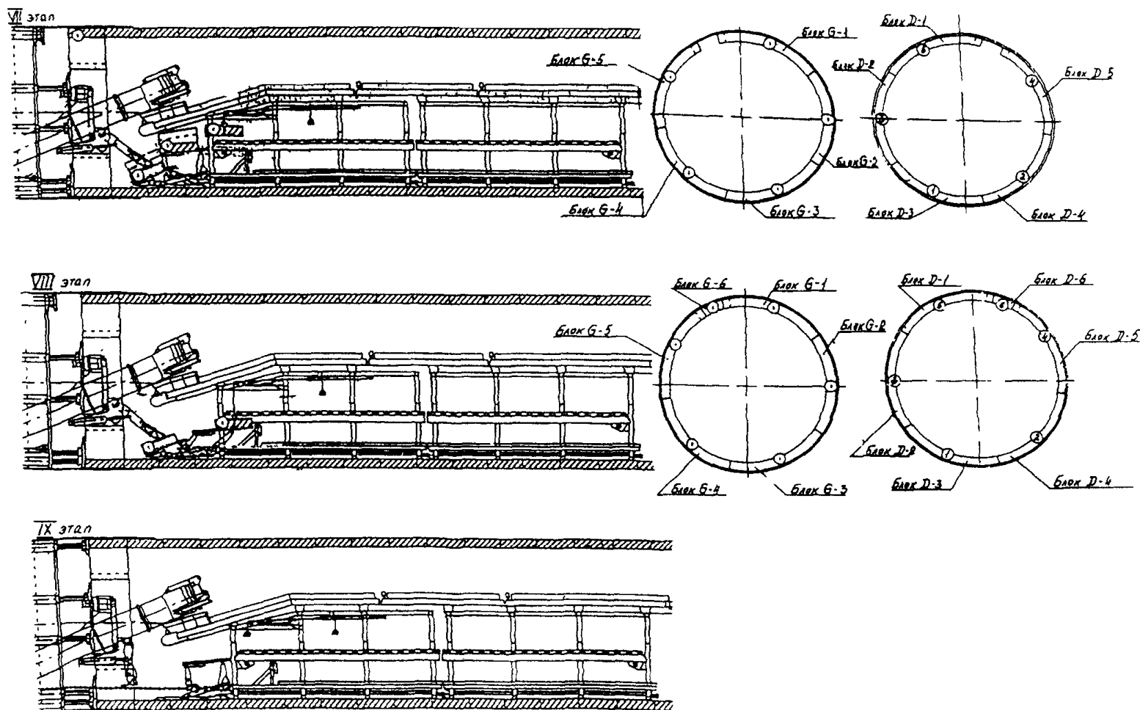
Рис. 8. Последовательность сборки кольца обделки тоннеля. Этапы VII, VIII, IX
