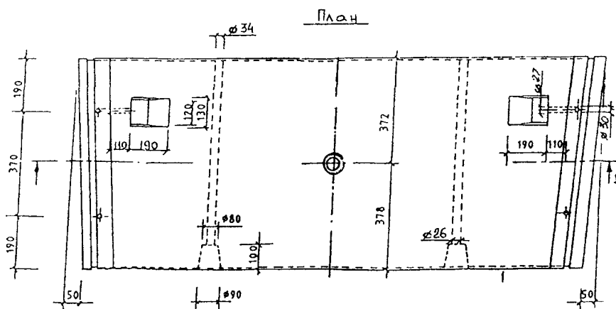
Рис. 3. Железобетонный блок обделки для коллекторных тоннелей внешним диаметром 4,0 м
