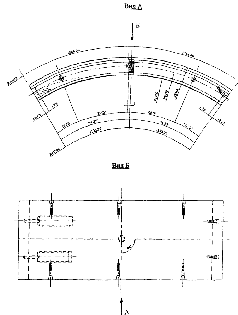
Рис. 2. Железобетонный блок обделки для коллекторных тоннелей внешним диаметром 4,36 м
