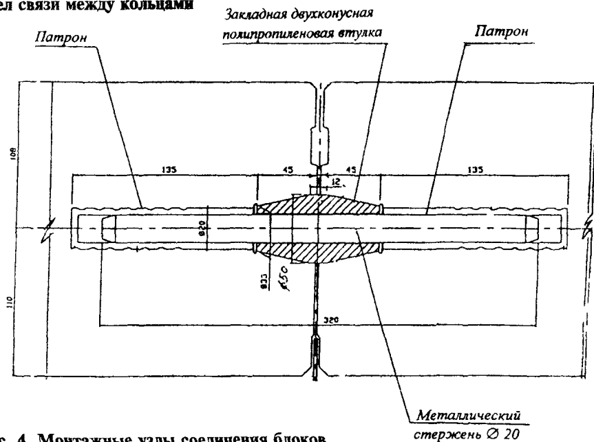
Рис. 4. Монтажные узлы соединения блоков
