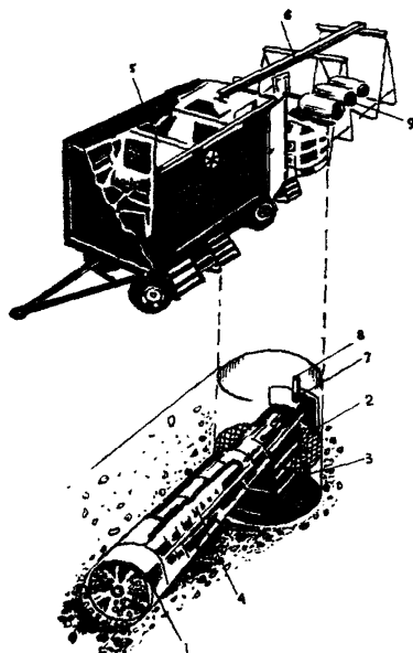
Рис.11. Конструктивно-технологическая схема МТПК 3-го вида (фирма "Зольтау") с щнековой транспортировкой разработанной породы:
