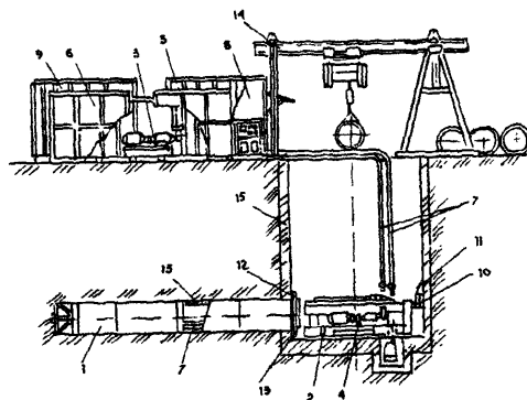
Рис. В1 Конструкторско-технологическая схема микротоннелепроходческого комплекса КМП-800 (проект ОАО НТЦ):
