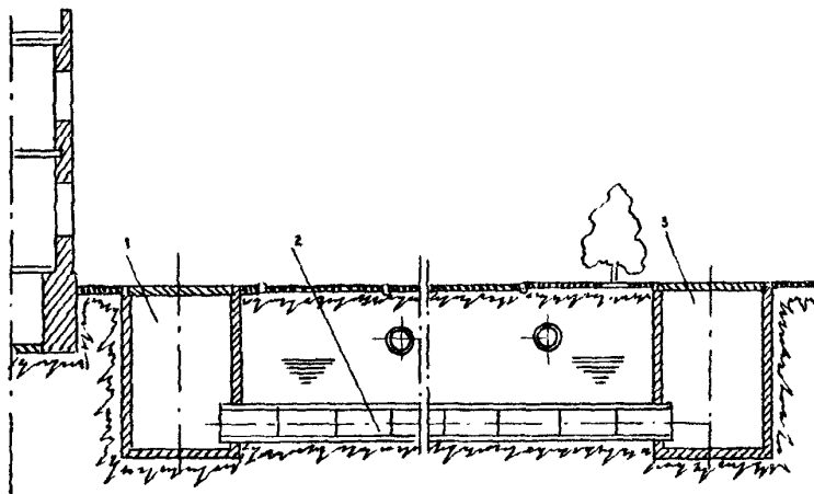
Рис.1. Схема трубопровода, проложенного бестраншейным способом между стартовой и конечной шахтами: 1—стартовая шахта; 2—трубопровод; 3—конечная шахта
