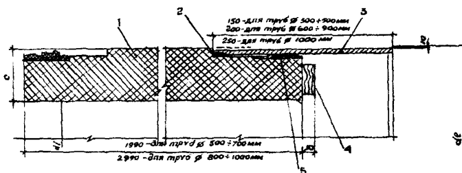
Рис.3. Стыковое соединение полимербетонных труб: 1-полимербетонная труба типа ТПБ; 2-герметик Тиксопрол-АМ марки 01 (ТУ 5712-004-18009705-95); 3- муфта соединительная типа МСМ; 4-кольцо компенсационное типа КК; 5-уплотнитель УП-40 для труб диаметром 300-500 мм УП-60-для труб диаметром 600-900 мм УП-40 (2 шт.)- для труб диаметром 1000 мм.
