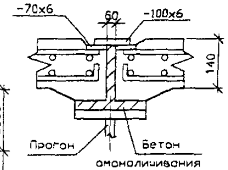
Деталь продольного шва плит М1:10
