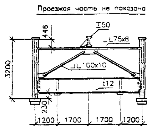
1-1 (повернуто) М1:100
