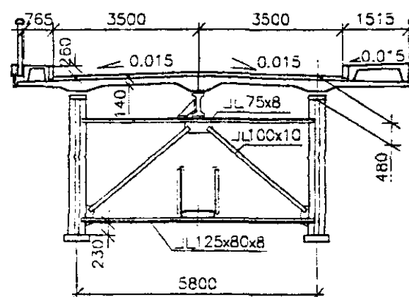
2-2 (повернуто) М1:100
