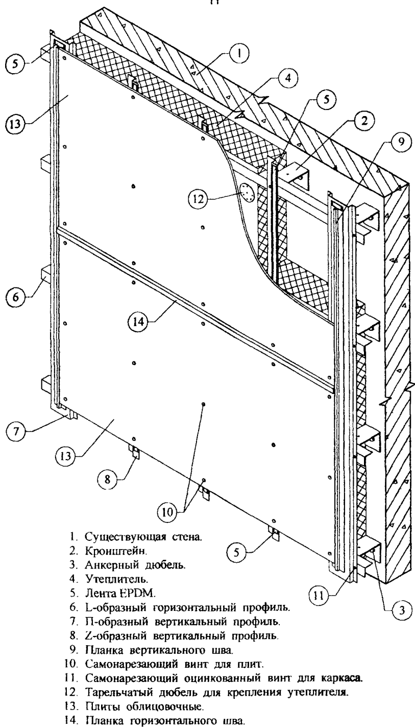
Рис. 3.1. Фасадная система "СЕМ-СИСТЕМА" с горизонтальным расположением плит.
