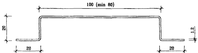
Рис. 3.4. Несущие вертикальные и горизонтальные профили (поперечное сечение).
